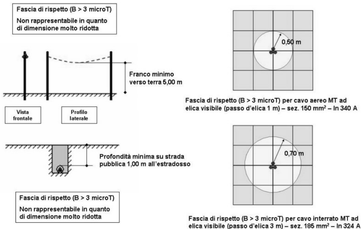
Fig. 1a Curve di equilivello per il campo magnetico di una linea interrata in MT con cavo elicordato (rif. Norma CEI 106-11)
