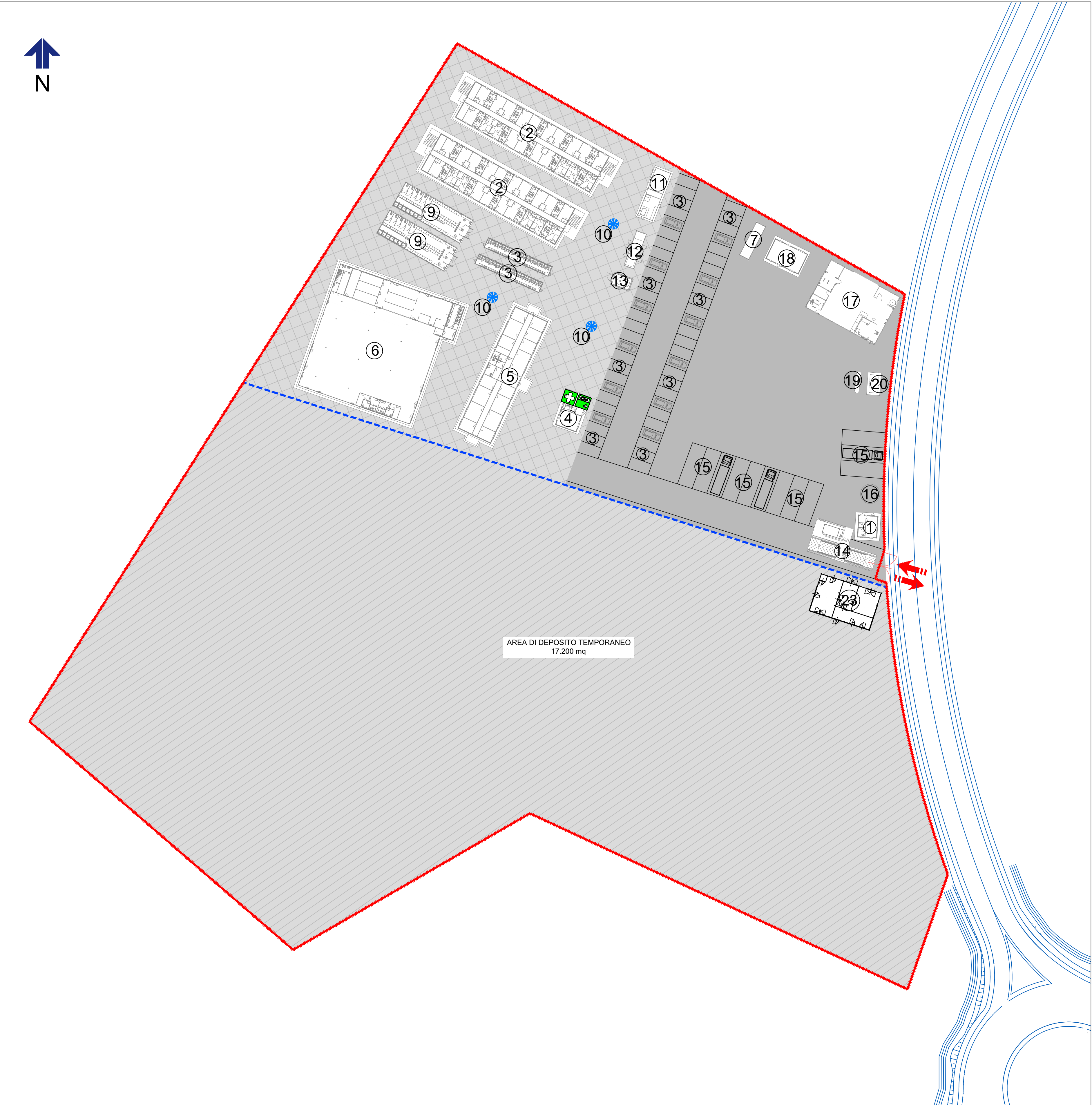
LAYOUT DI CANTIERE 1:500
