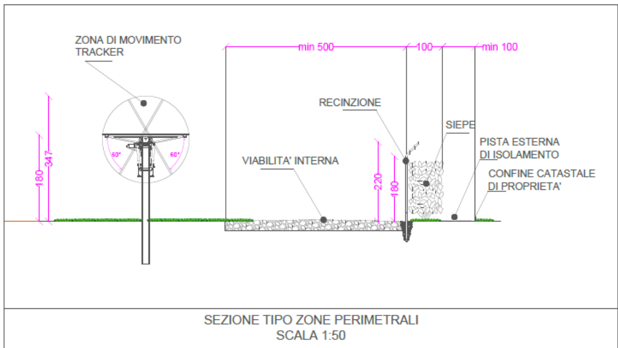
Figura 16 - elaborato A.12.c.1 (DISEGNI ARCHITETTONICI Recinzione tipo impianto fotovoltaico)
