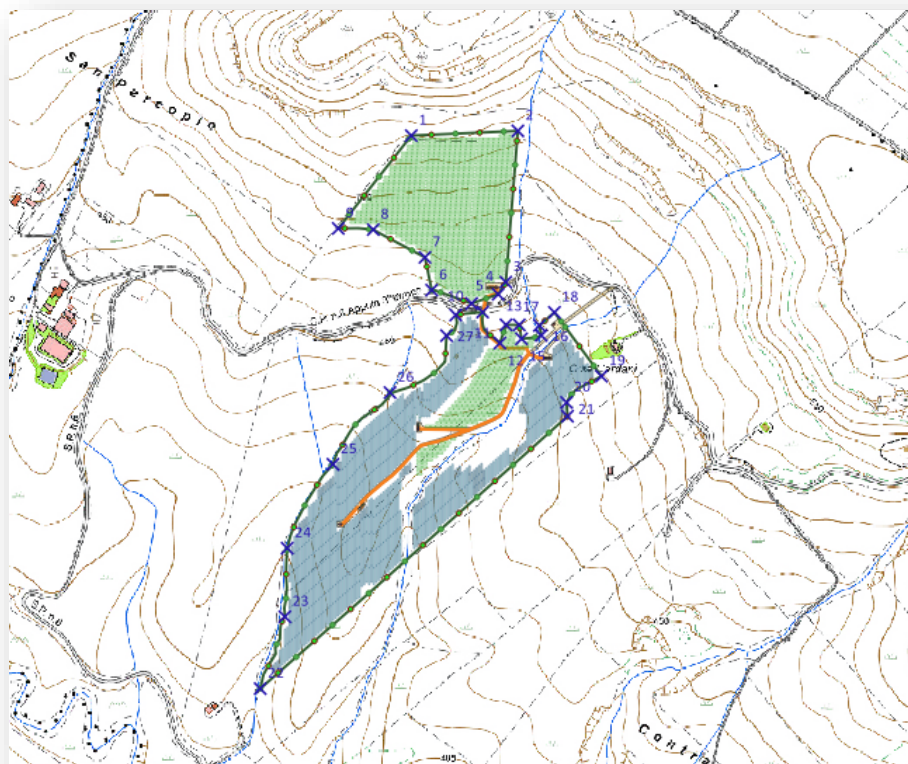
Figura 1 - Rappresentazione grafica aree occupate dell'impianto
