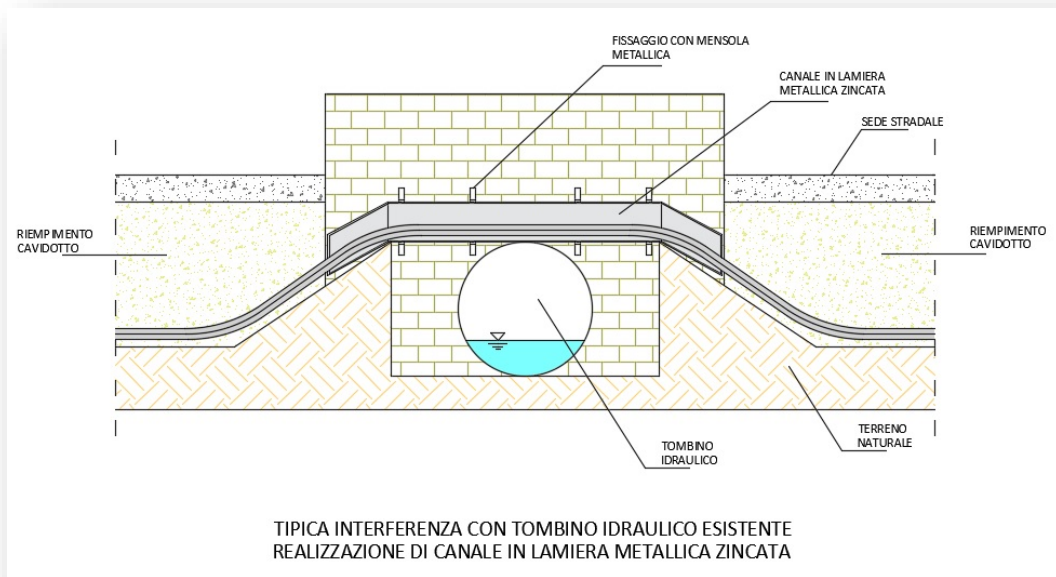
Figura 25 - schema tipico di risoluzione interferenza con tombino idraulico mediante realizzazione di canale in lamiera metallica zincata (staffaggio esterno)
