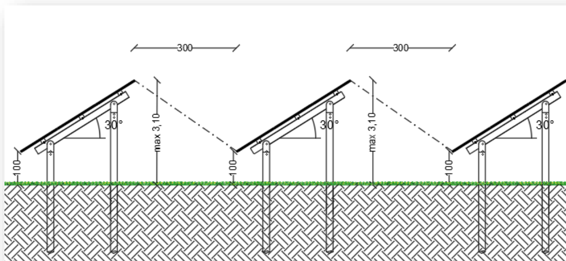
Figura 11 – Sezione tipo impianto nella configurazione fissa.
