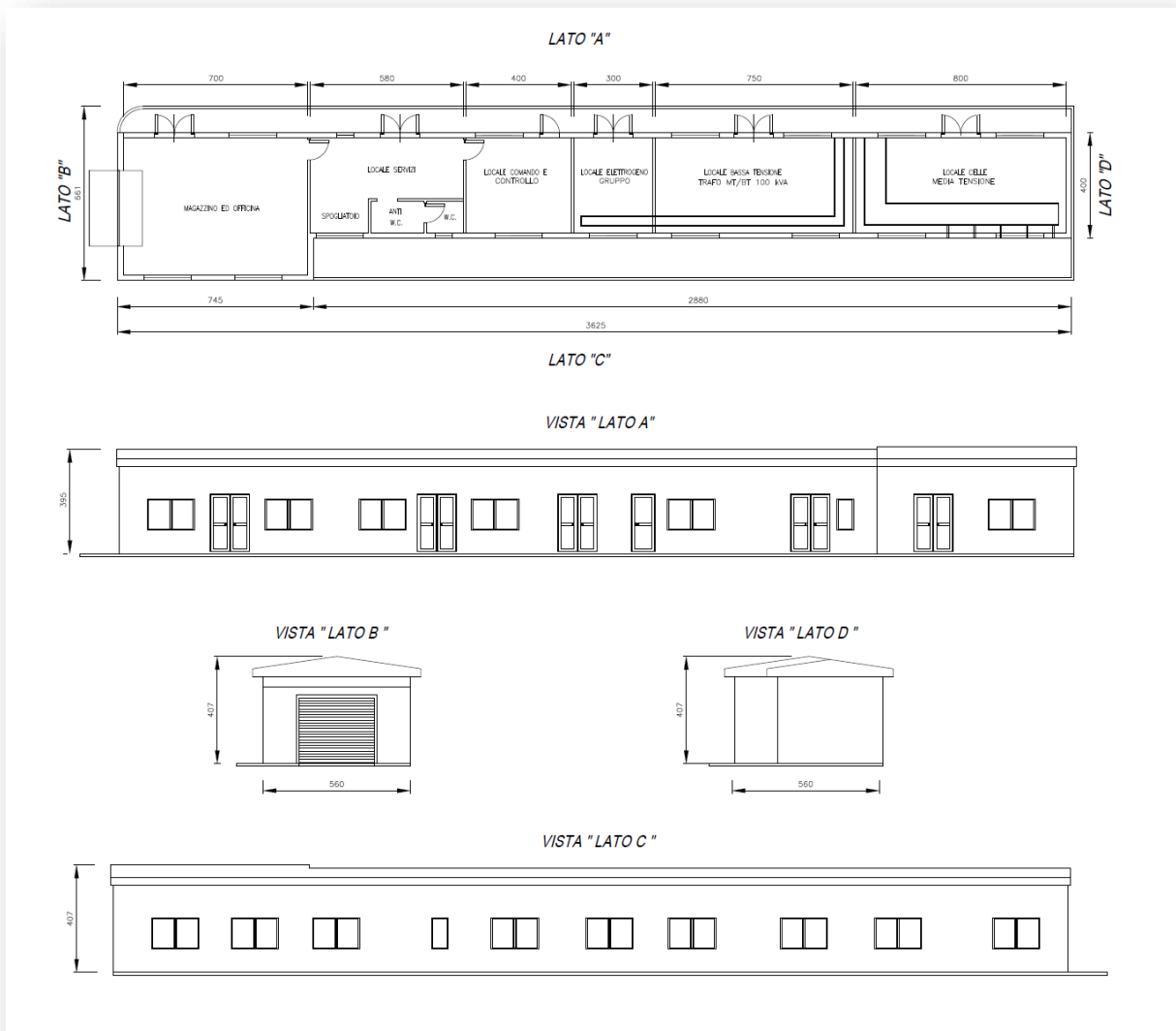
Figura 12 - Estratto elaborato A.12.b.10.a (Edificio di controllo SSE)
