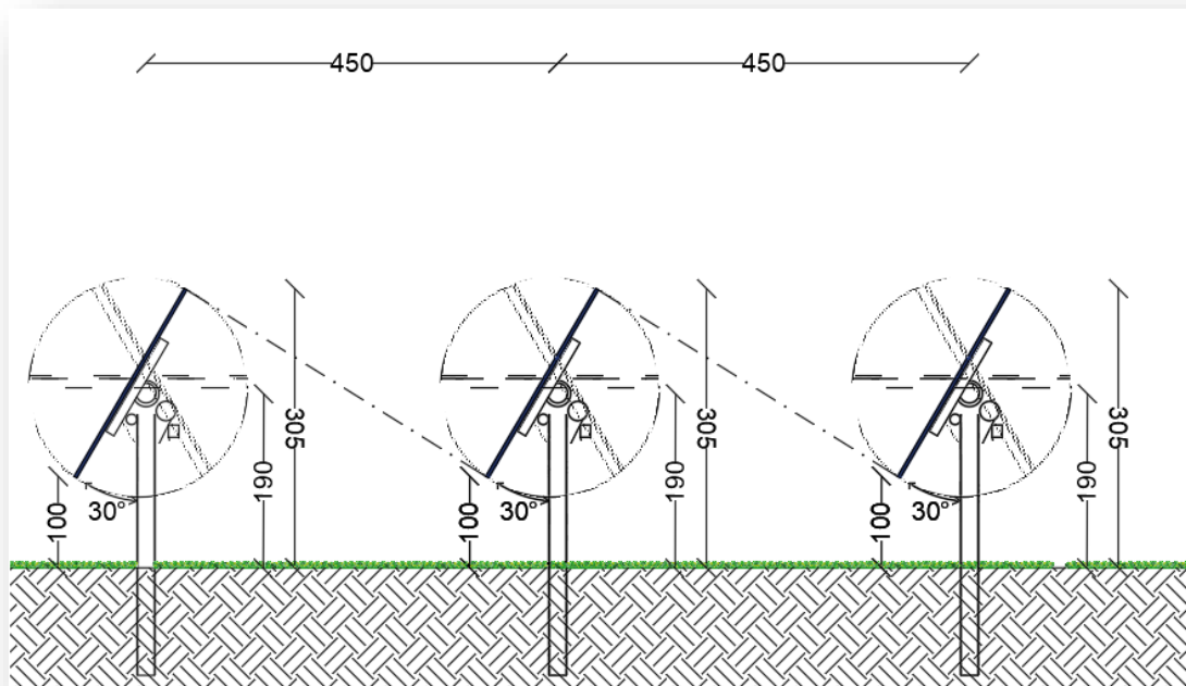
Figura 10 – Sezione tipo impianto nella configurazione tracker
