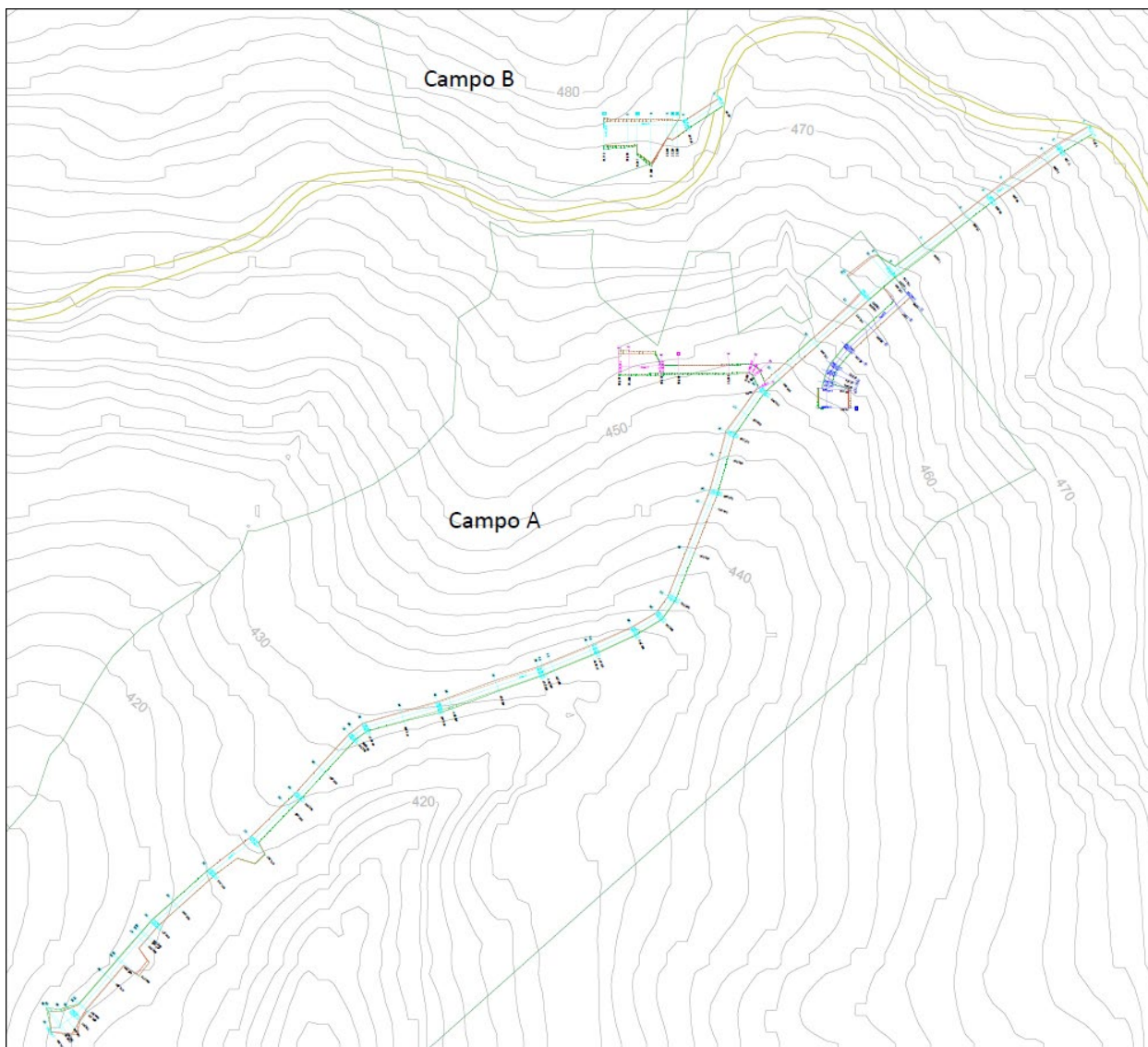
Figura 20 - Estratto della tavola A.12.a.13 – Planimetria Viabilità interna al parco
