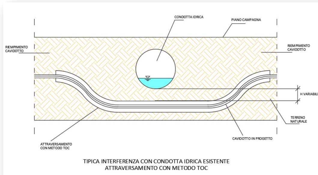
Figura 27 - schema tipico di risoluzione interferenza con condotte idriche esistenti mediante l'utilizzo di metodo TOC
