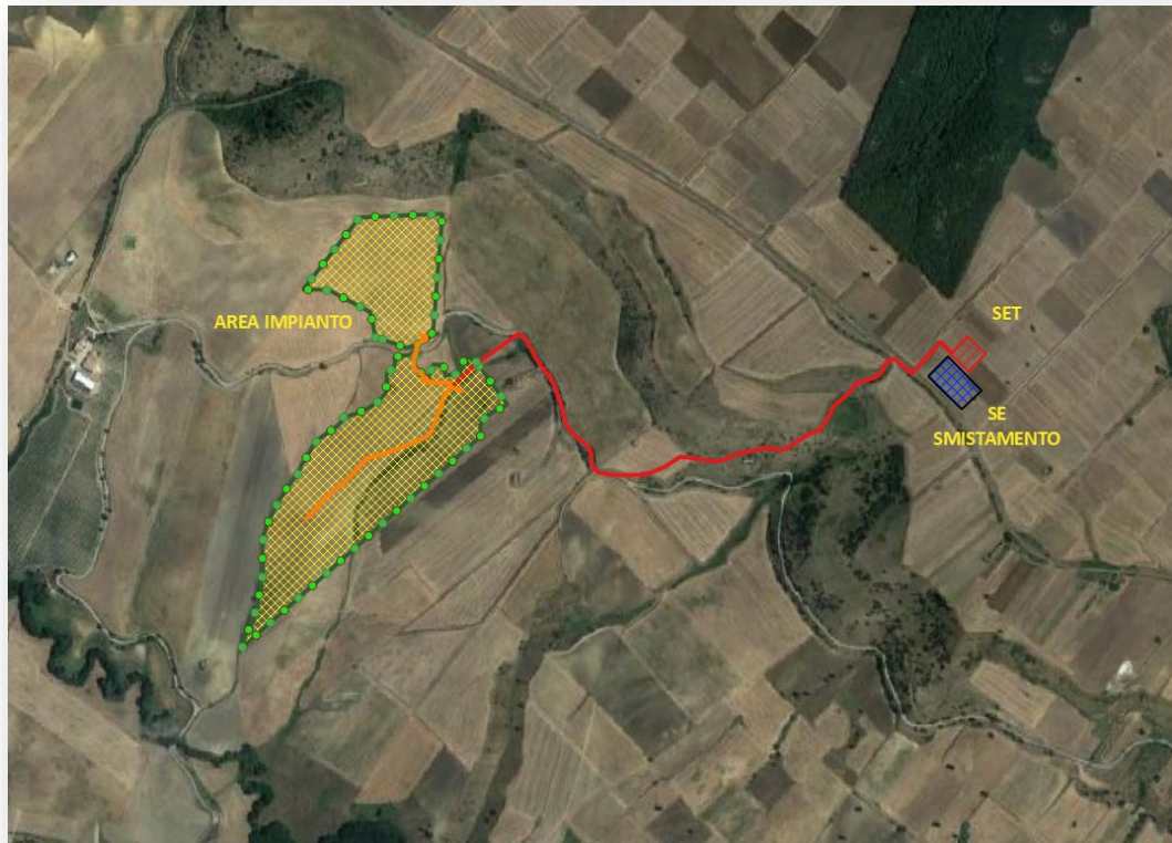
Figura 2- Percorso dell'elettrodotto interrato MT da realizzare (tratto in rosso)
