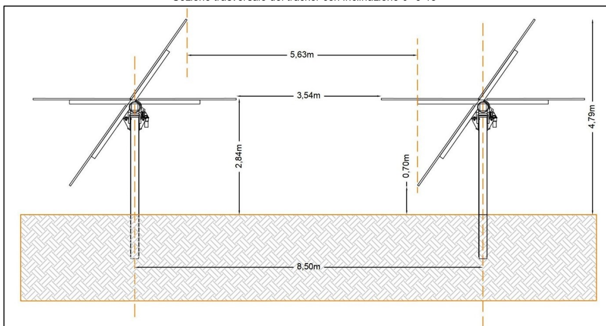
Figura 3.1. Prospetto trasversale e longitudinale delle strutture da installare
