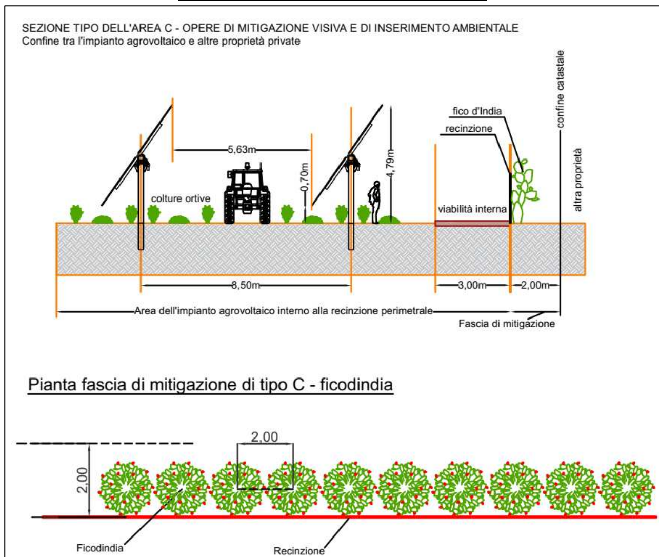
Figura 6.2-C. Fascia di mitigazione di tipo C (ficodindia)
