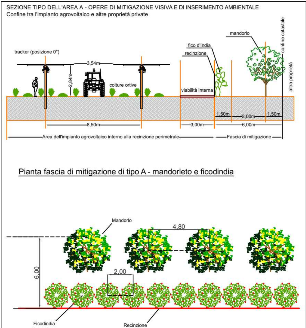
Figura 6.2-A. Fascia di mitigazione di tipo A (Mandorlo-ficodindia)
