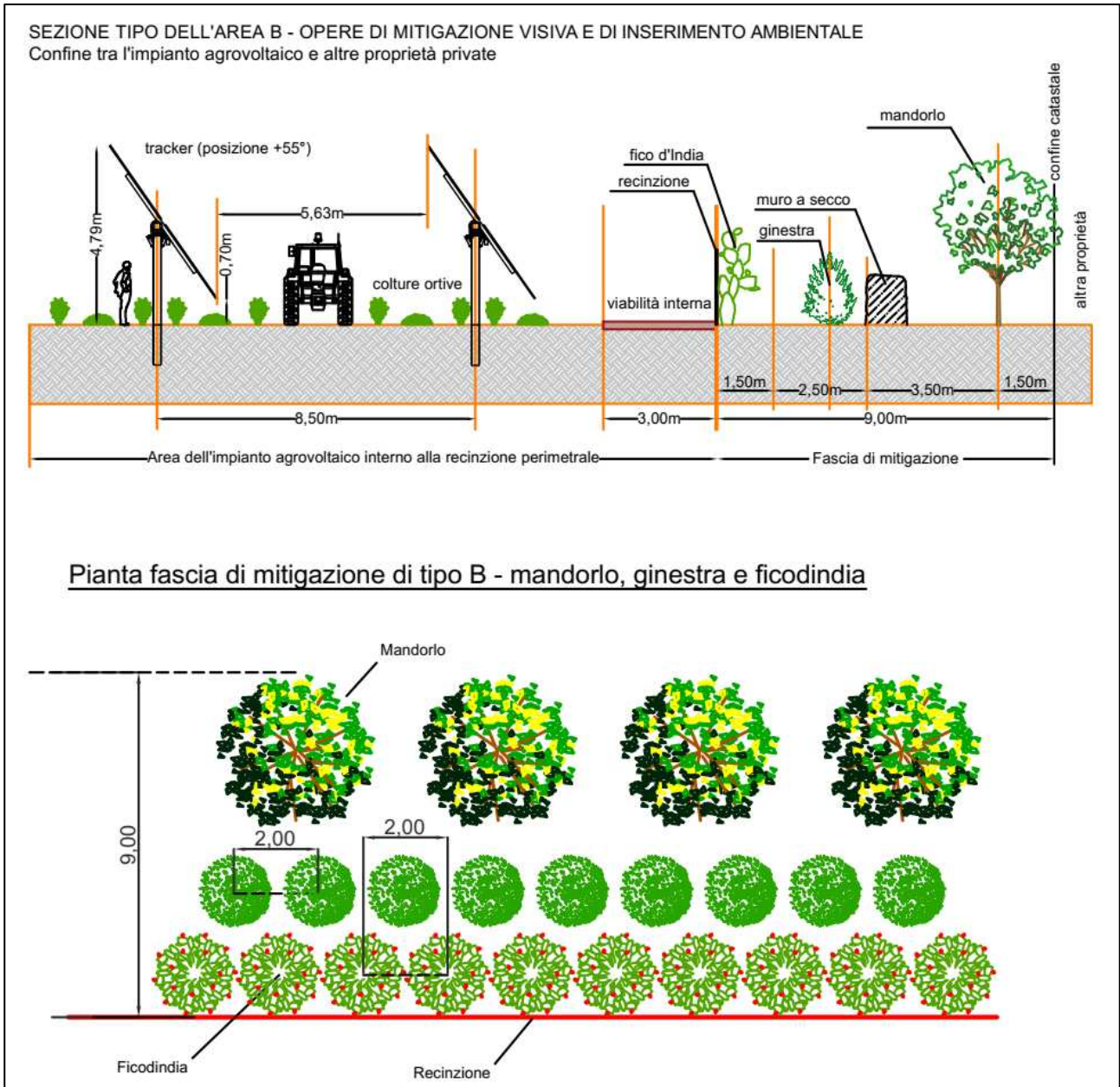
Figura 6.2-B. Fascia di mitigazione di tipo B (Mandorlo, ficodindia e piante arbustive autoctone)
