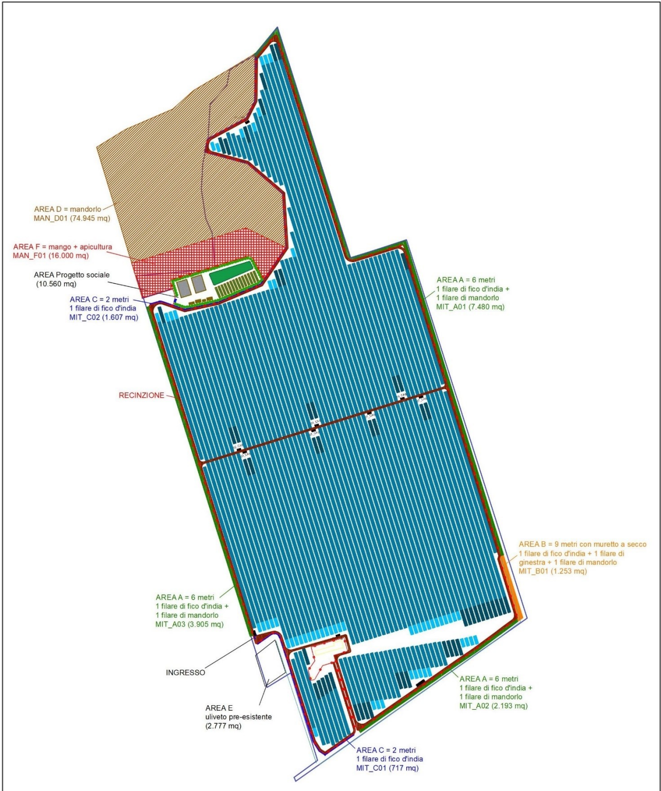
Figura 6.1. Sagome delle superfici indicate alle tabelle precedenti
