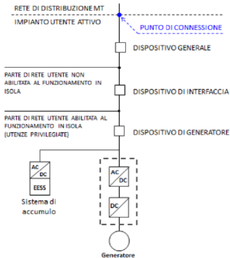
Figura 2 Connessione alla rete dell’impianto BESS come da CEI0-16
