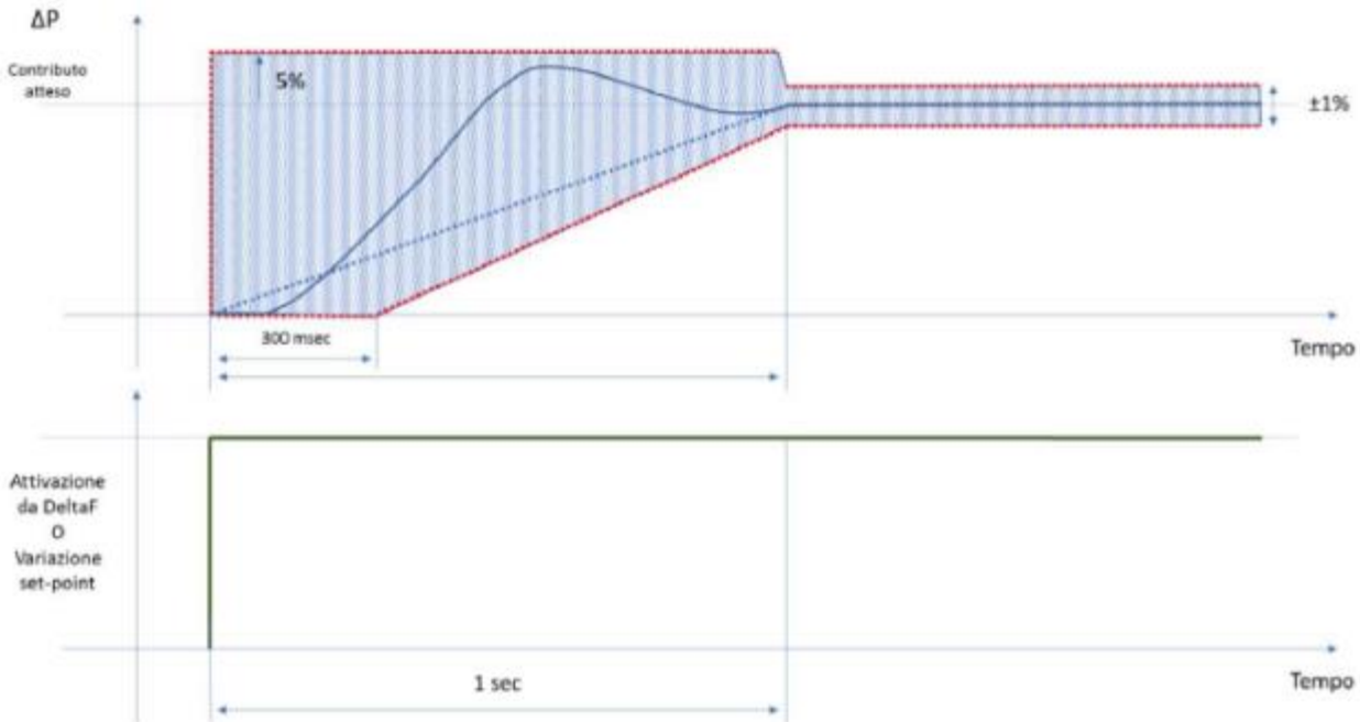
Figura 4 Requisiti Fast Reserve: Rampa e precisione statica e dinamica
