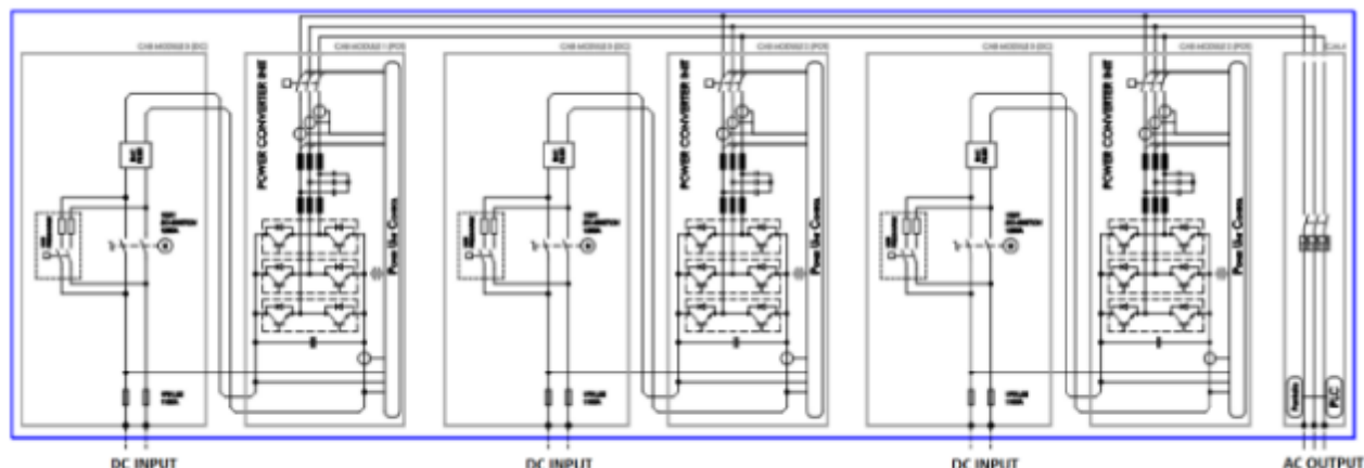
Figura 3 Schema Unifilare dell’inverter
