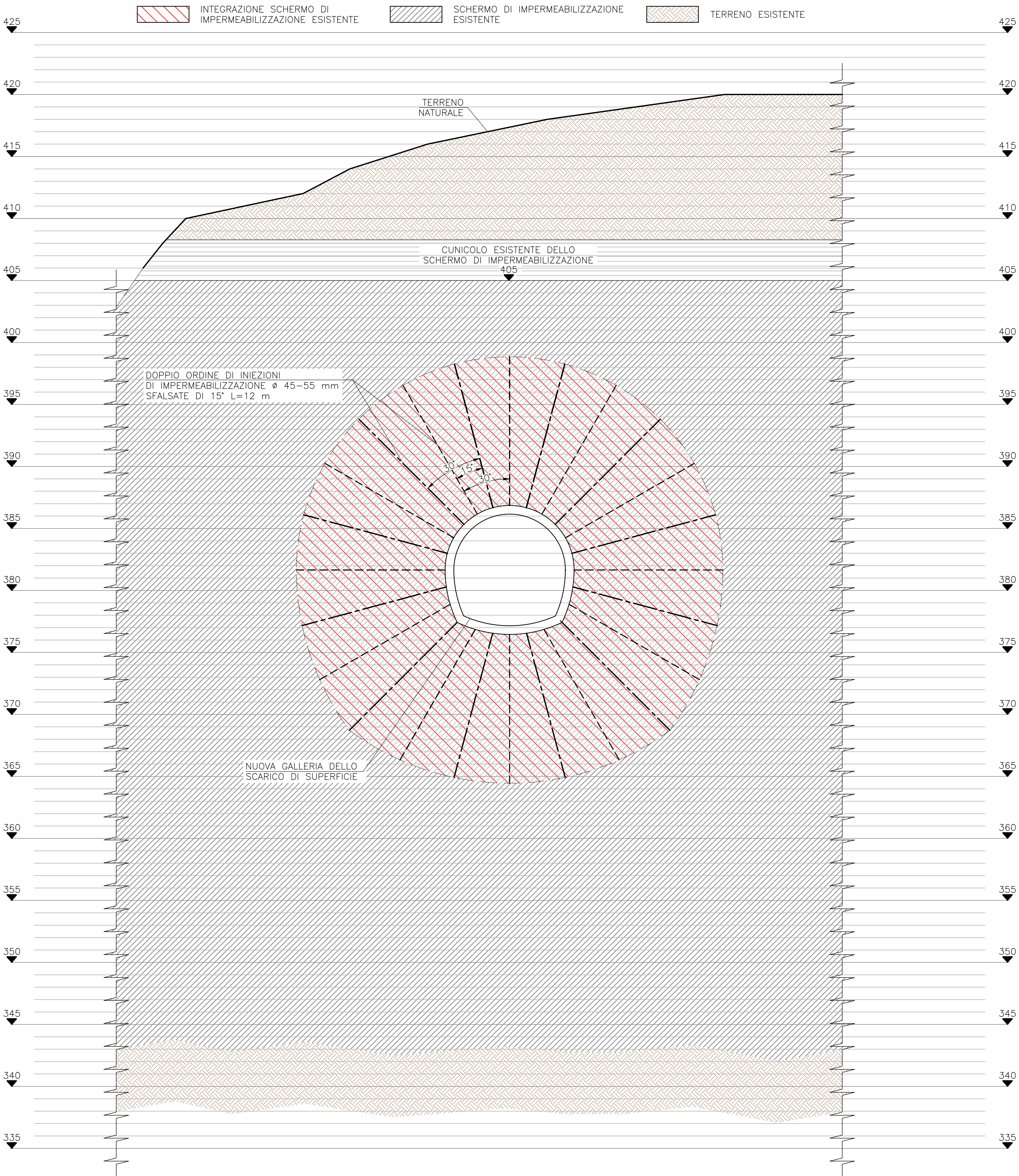
SEZIONE DELLA GALLERIA IN CORRISPONDENZA DELLA PROGRESSIVA 66.06 SCALA 1:200
