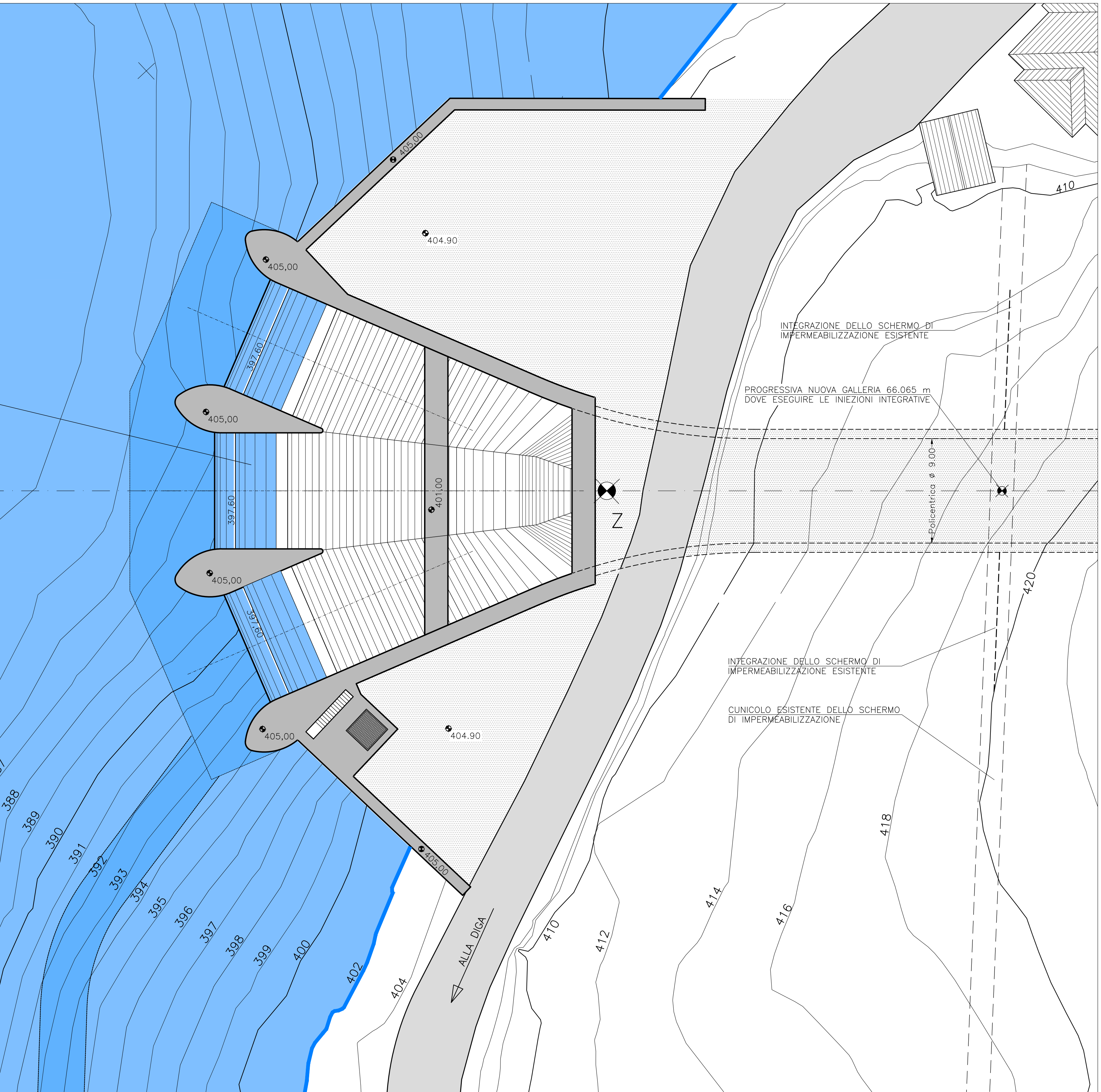
PLANIMETRIA DI DETTAGLIO SCALA 1:200
