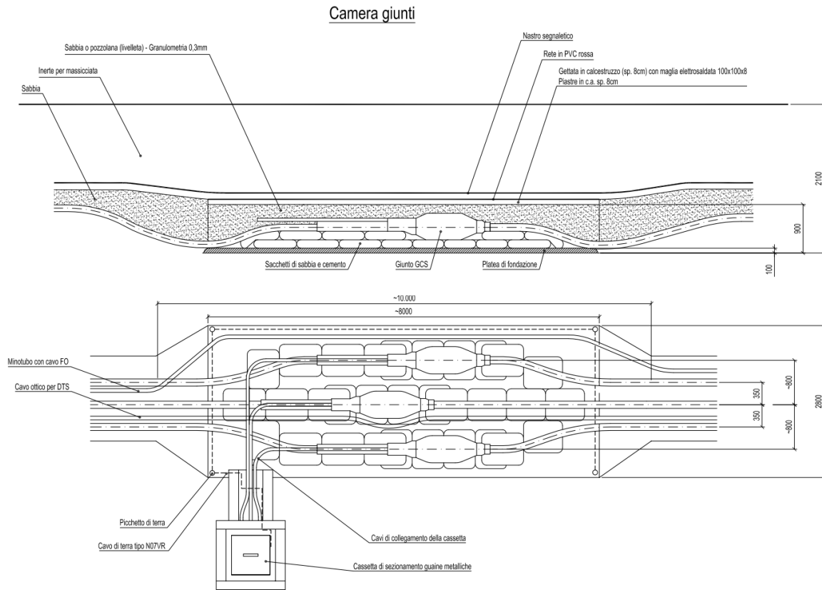
Esempio tipologico buca giunti terrestre
