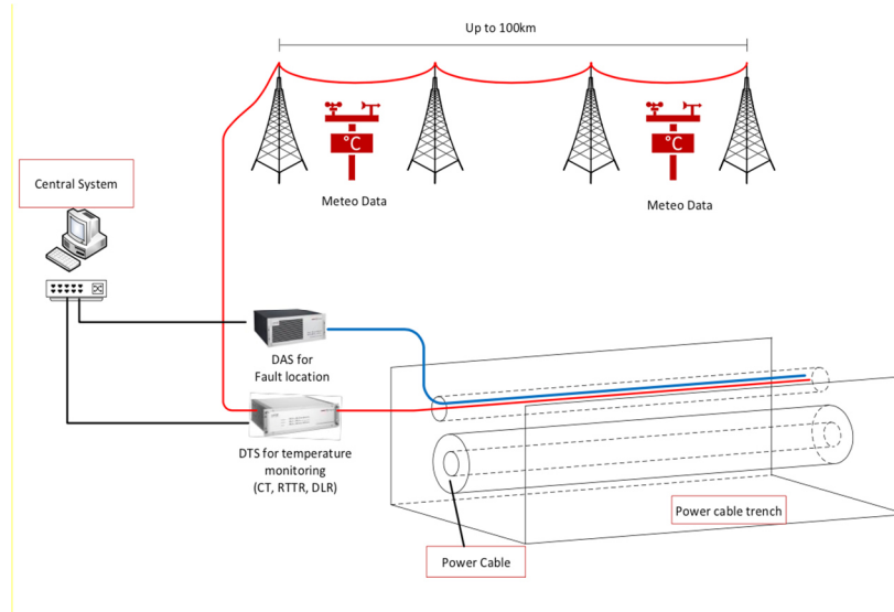
Esempio di sistema per monitoraggio della sezione in cavo tramite DTS/DAS per cavi interrati
