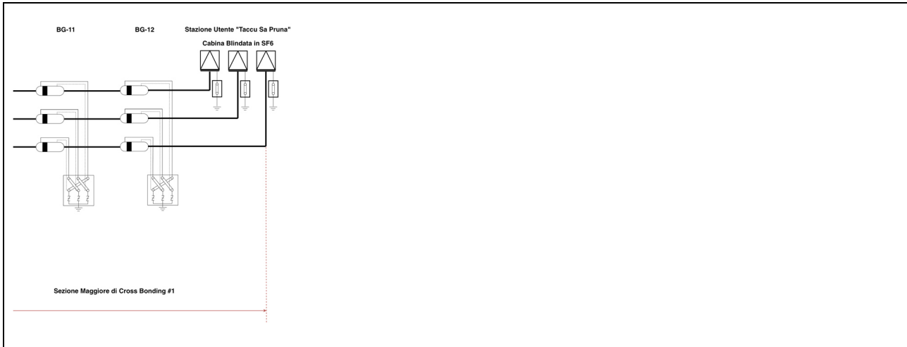
Sistema di connessione delle guaine Tratta Giunto di transizione cavo in galleria - Terminali Trasformatore Stazione Utente "SU Villarosa"
