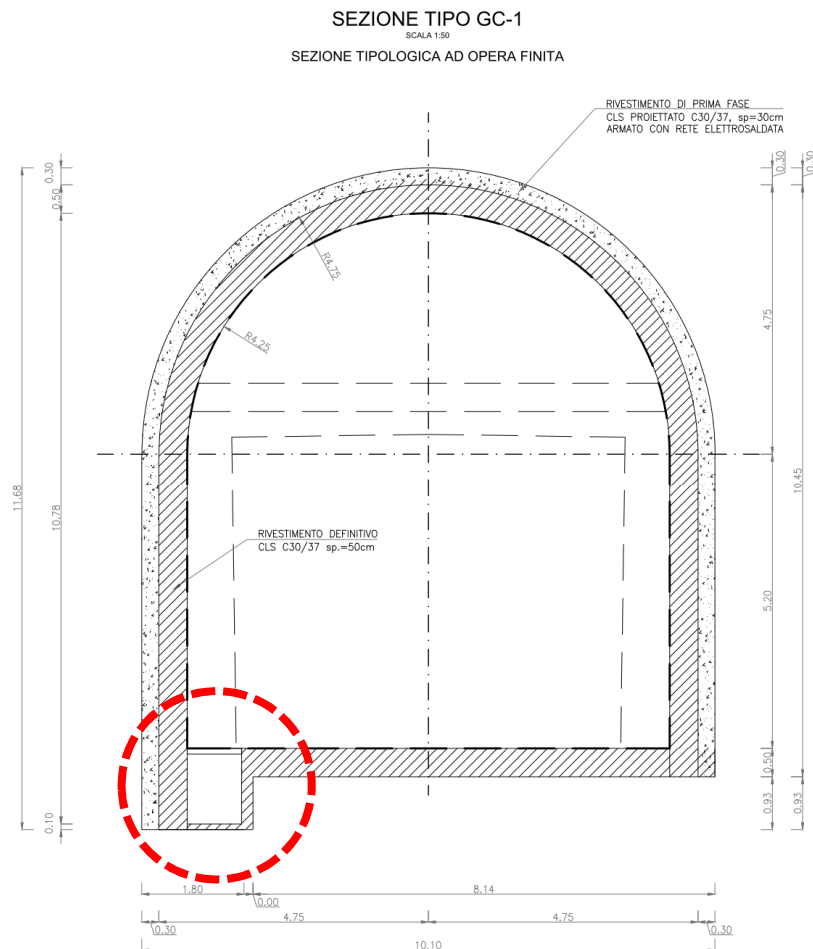
Sezione tipologica galleria di accesso alla centrale in caverna con indicato il cunicolo per i cavi AT
