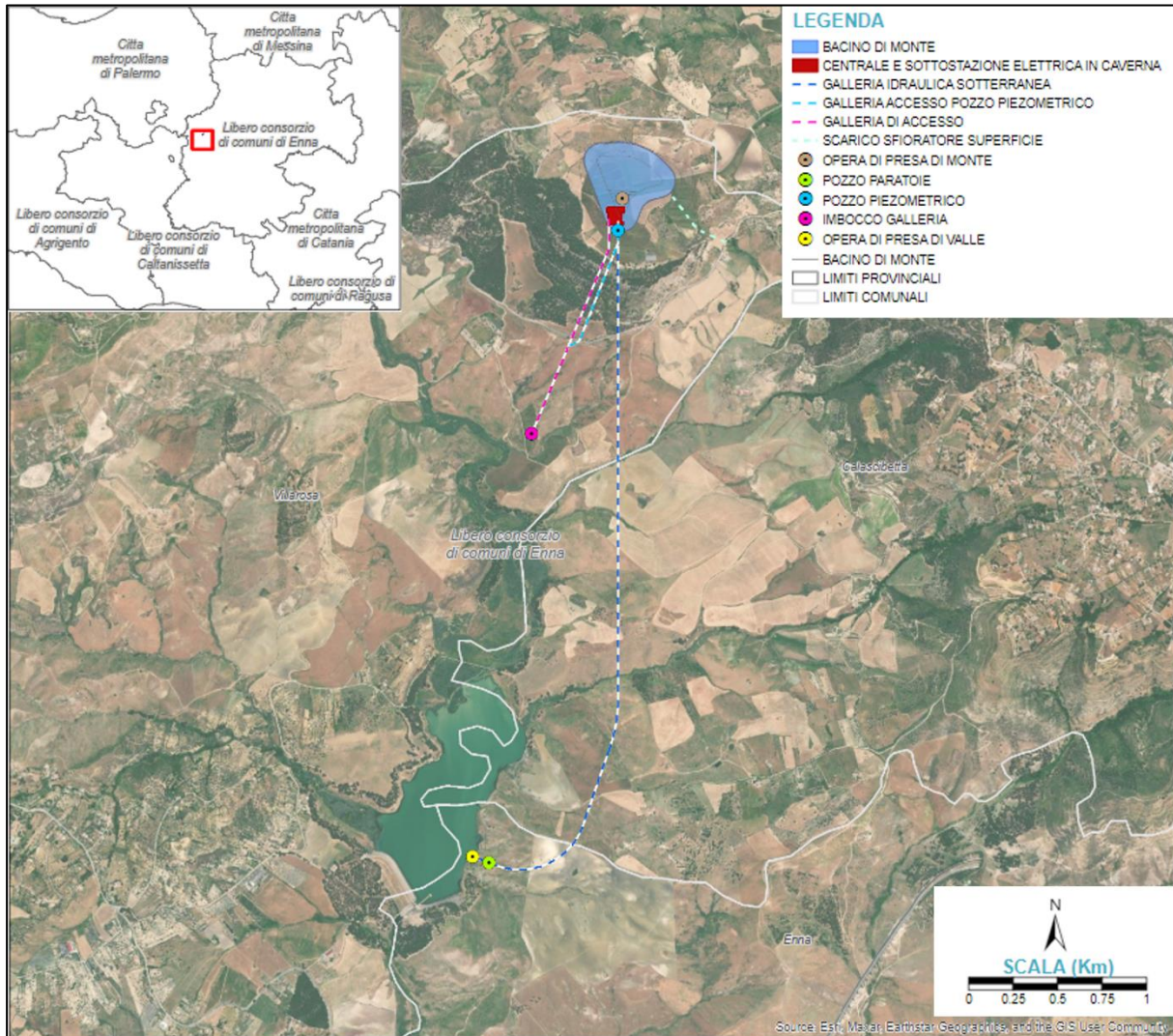
Figura 2.1: Ubicazione dell’Impianto di Accumulo Idroelettrico di Villarosa
