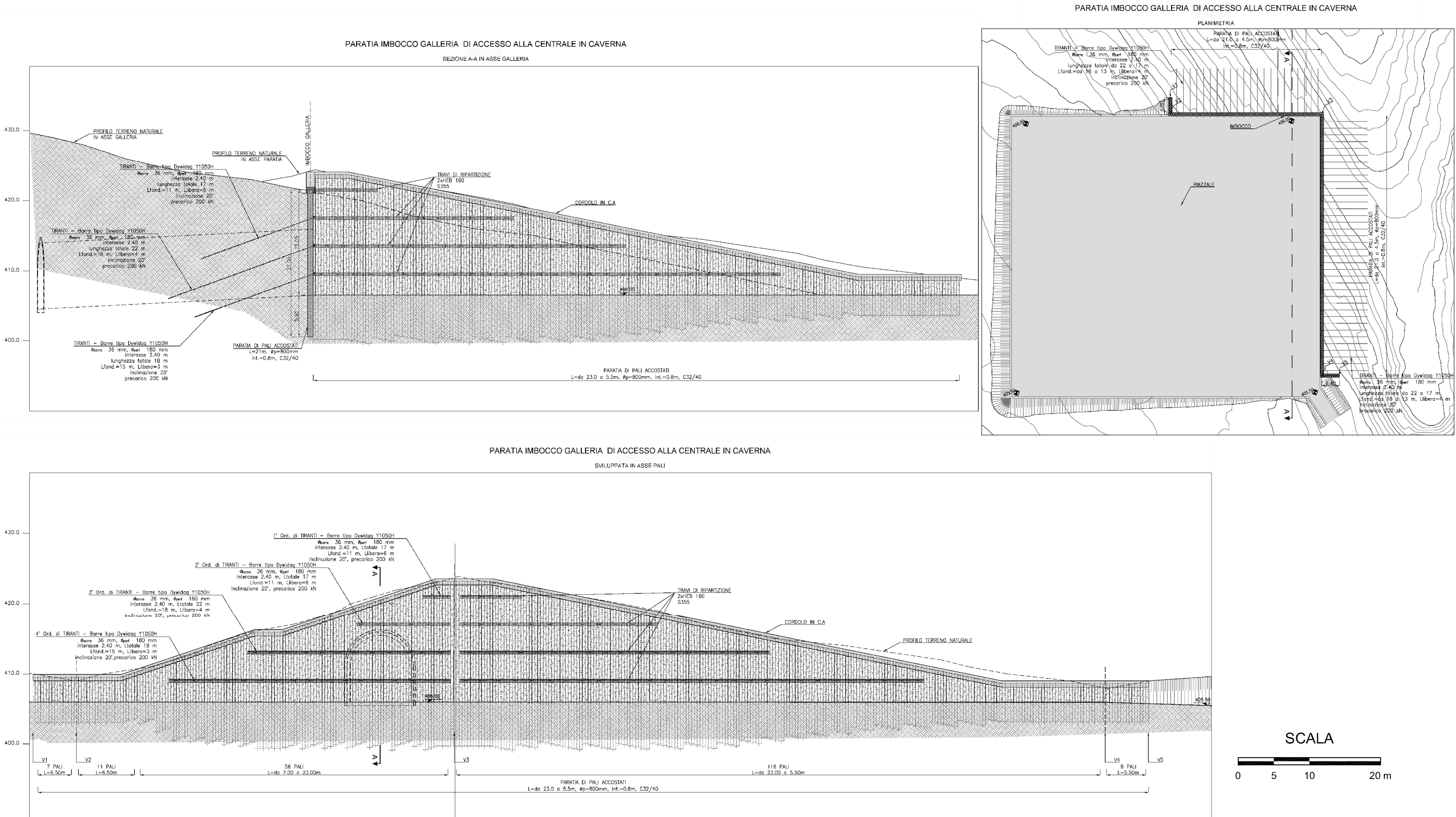
FIGURA 3.3 FINESTRA D'ACCESSO OPERE SOTTERANEE - OPERA DI IMBOCCO
