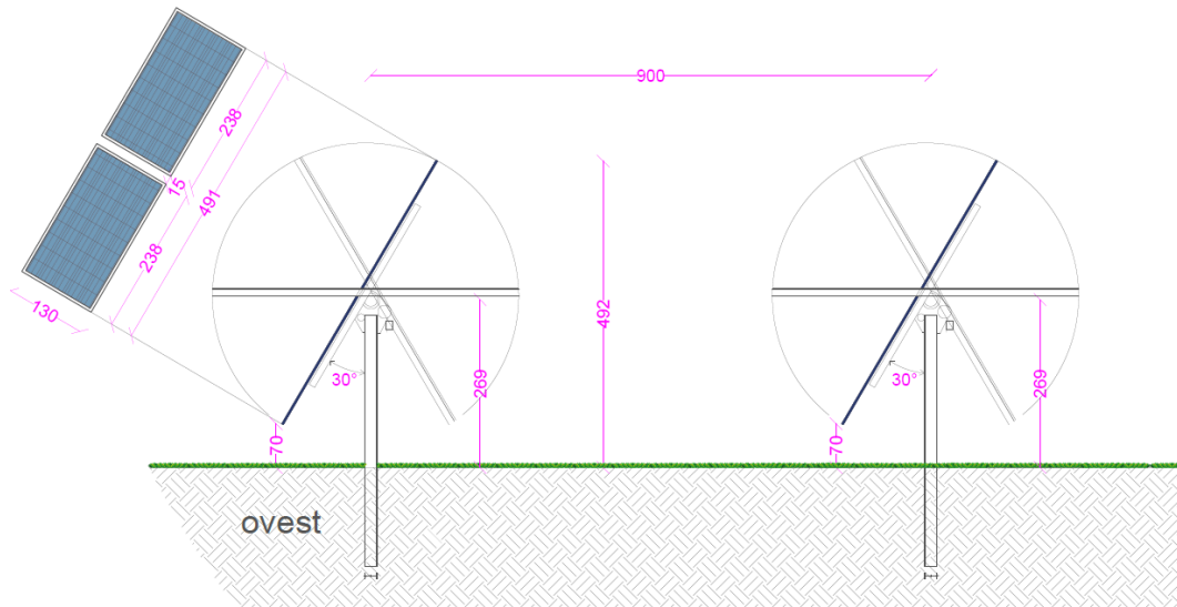
Figura 2 – Sezione tipo impianto nella configurazione tracker
