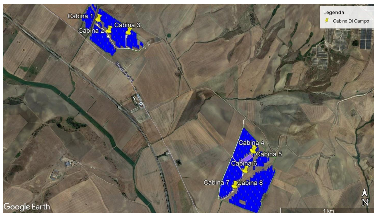
Figura 9 – Cabine di Campo
