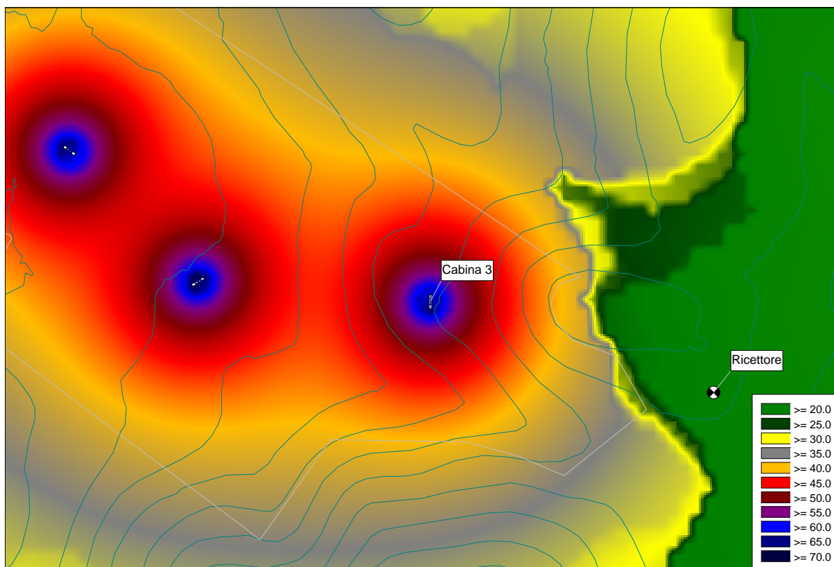
Figura 11 – Rappresentazione grafica mappa orizzontale di dettaglio con curve di isolivello decibel
