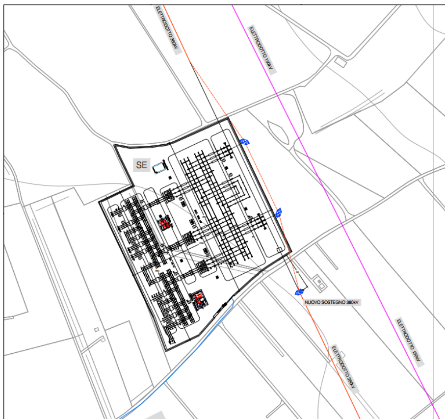
Figura 6: Layout dell'impianto
