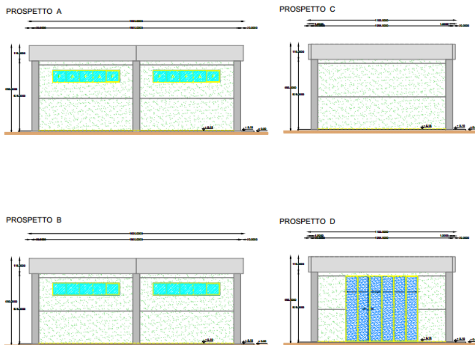
Figura 4: Prospetti edificio Magazzino
