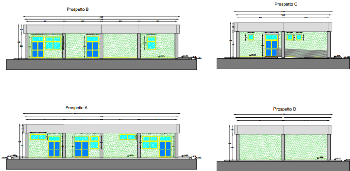
Figura 2: Prospetti edificio Comandi
