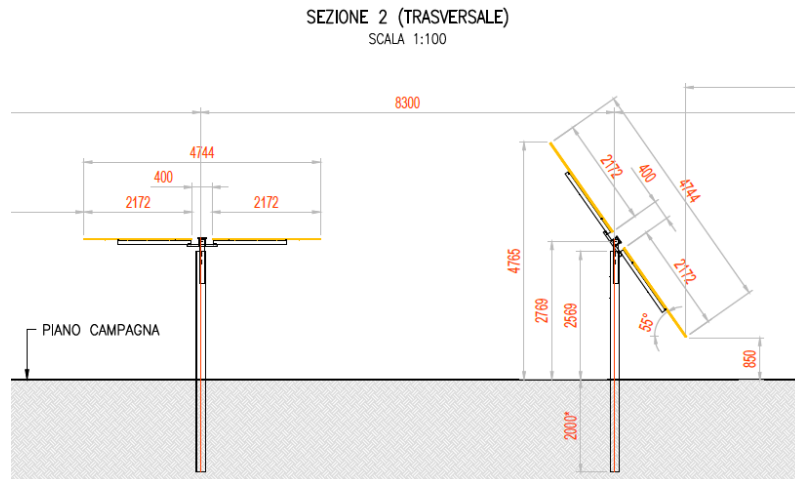
Figura 4.4: Particolare strutture di sostegno moduli
