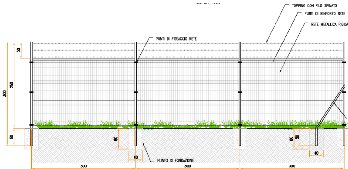
Figura 4.6: Particolare recinzione
