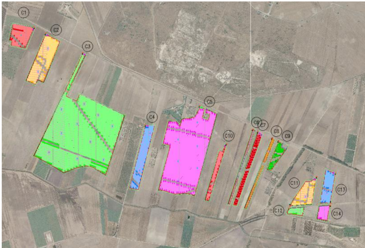
Figura 4.1: Layout di progetto
