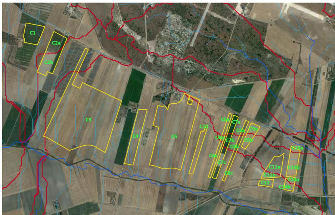
Figura 5.5: Delimitazione bacini scolanti e codifica (giallo), reticolo di drenaggio esterno ed interno alle sezioni di progetto (blu) e limiti dei bacini idrografici (rosso).
