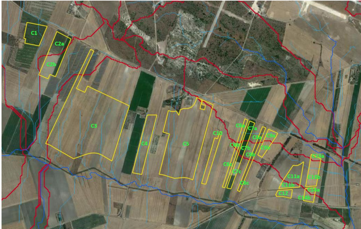
Figura 5.9: Delimitazione aree di impianto e rete di drenaggio naturale interna.
