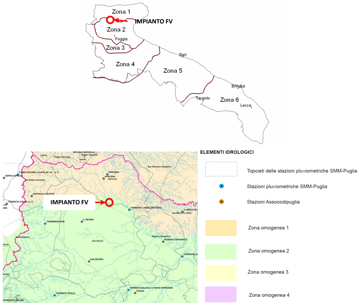
Figura 5.3: Sottostazioni pluviometriche omogenee ed ubicazione area di progetto.
