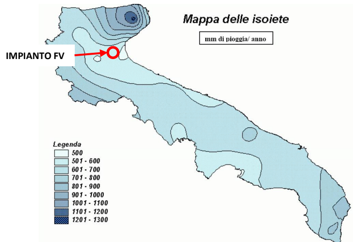
Figura 5.1: Mappa delle isoiete della Regione Puglia.
