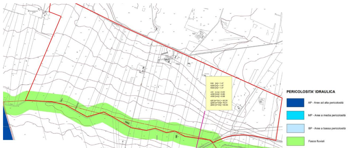
Figura 3.13: Stralcio carta di pericolosità idraulica nr. 100 “Foggia” e nr. 101 “Manfredonia” del PGRA aggiornata al 30/03/2016. In rosso l’area di progetto.
