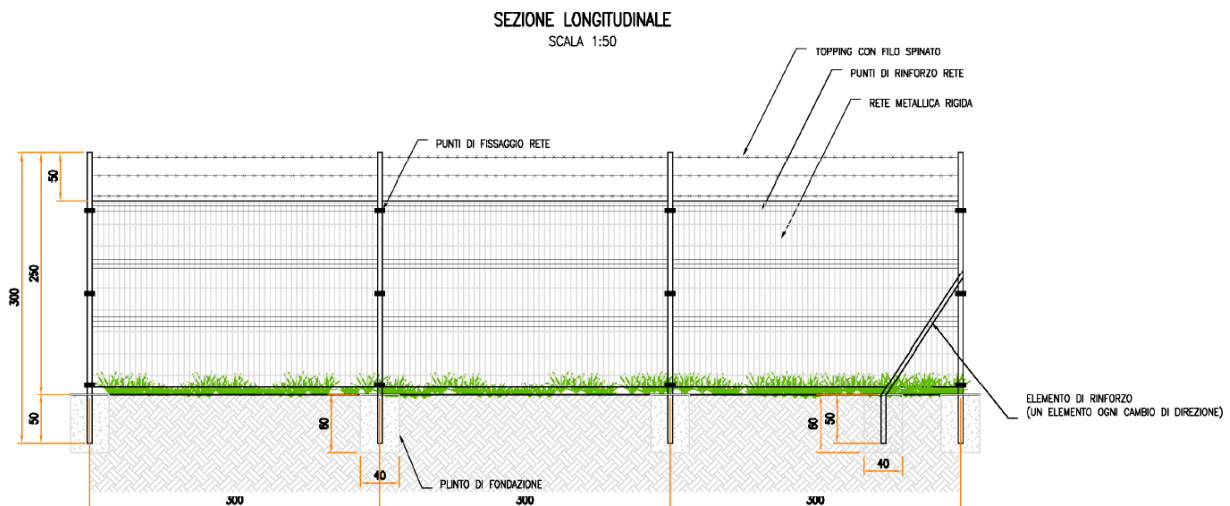
Figura 5.1: Tipico recinzione
