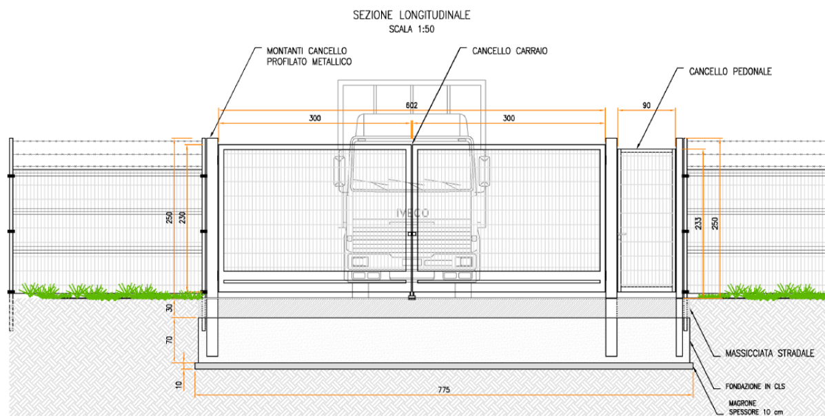
Figura 2.9: Particolare accesso
