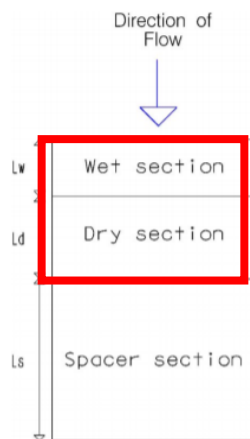
Figura 4.7: modulo tipo descrivente il modello concettuale idrologico dell'installazione di strutture fotovoltaiche a tracker su pari infissi comprendente l'area pannelli (in rosso) e l'area di interfila (Fonte: Hydrologic response of solar farm Cook 2013 American Society of Civil Engineers)
