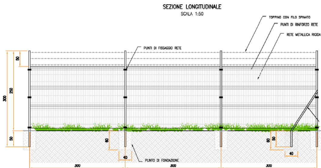
Figura 2.7: Particolare recinzione
