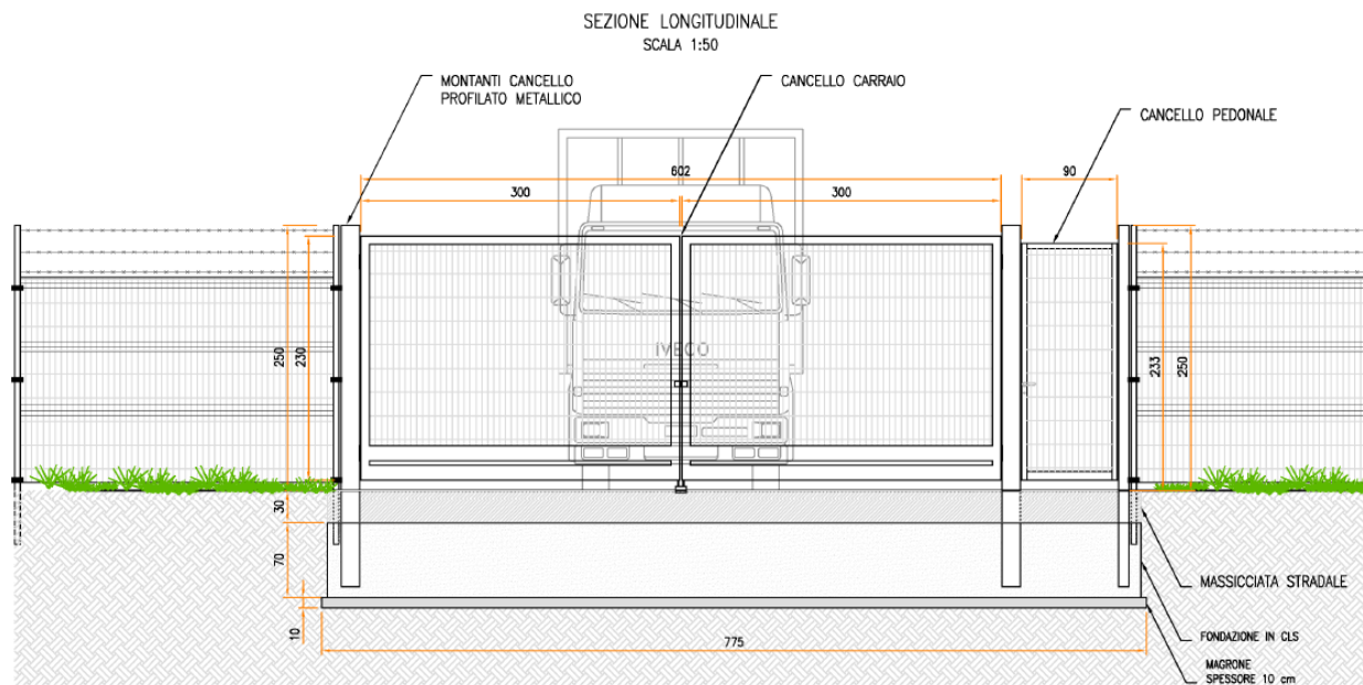
Figura 2.9: Particolare accesso
