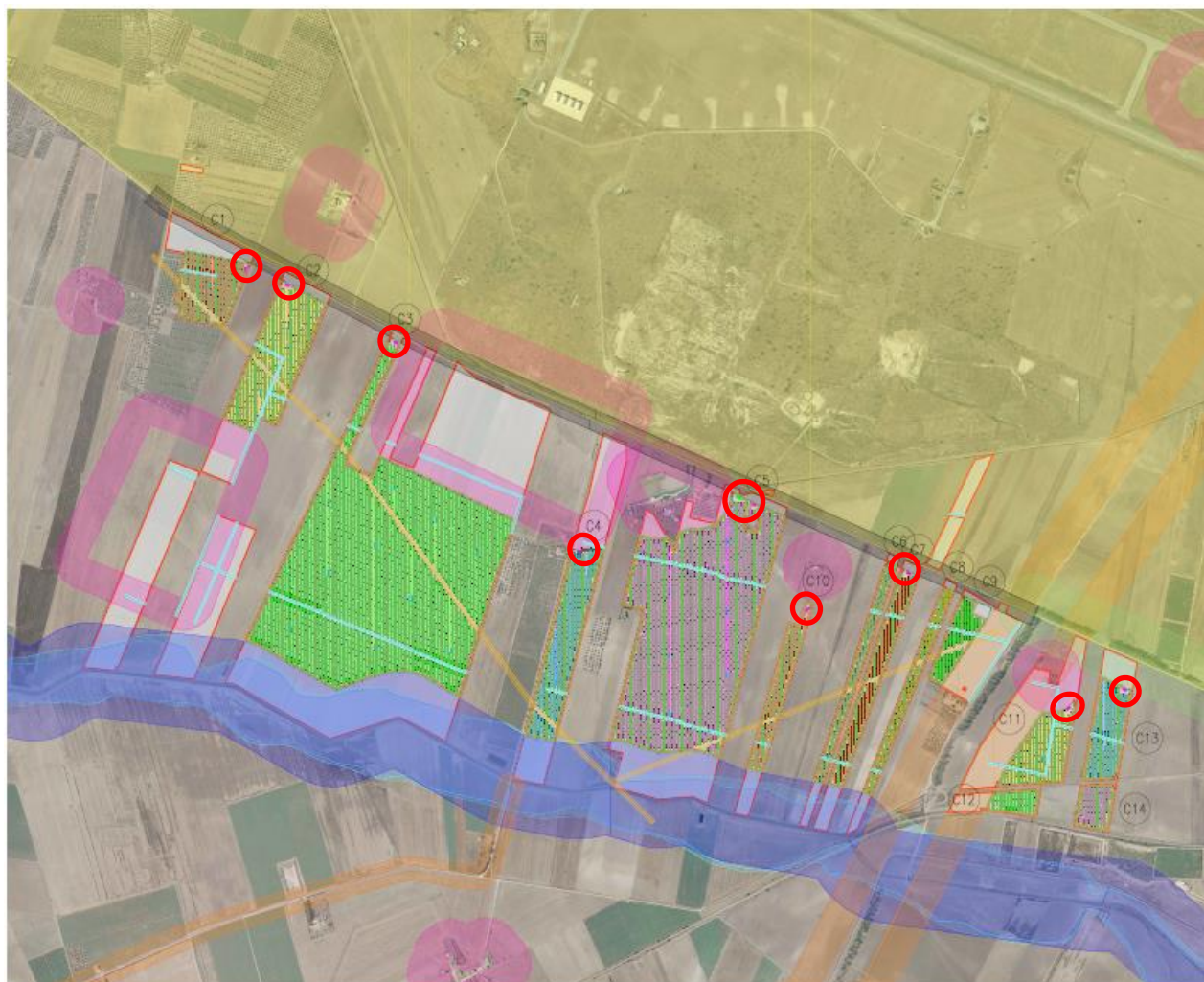
Figura 4.3: Spazi accessori dell'impianto (particolare delle tavole progettuali), in rosso
