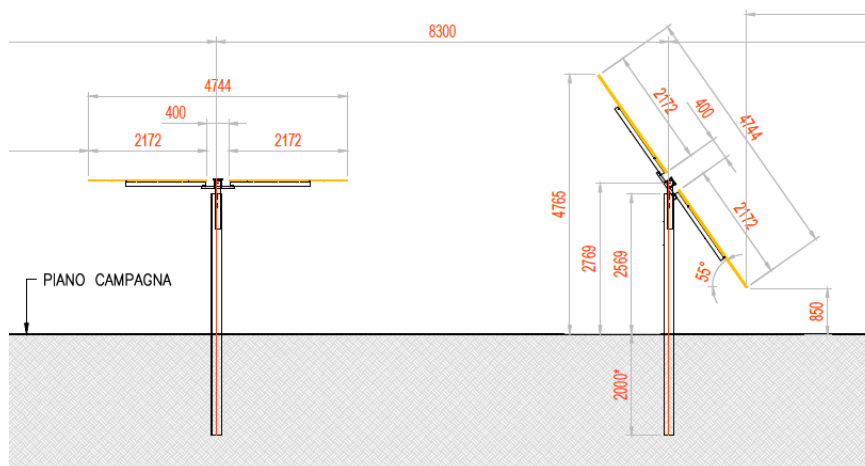
Figura 2.5: Particolare strutture di sostegno moduli
