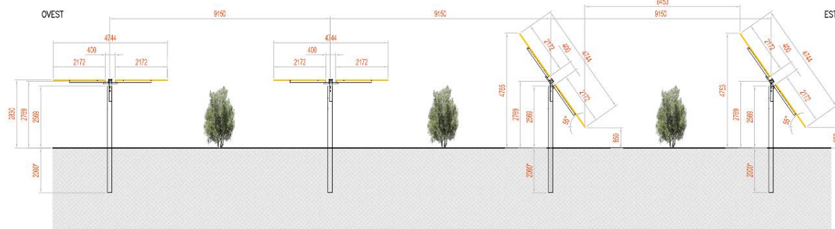
Figura 2.14: Tipologico – Vista in Sezione dell'impianto Olivicolo
