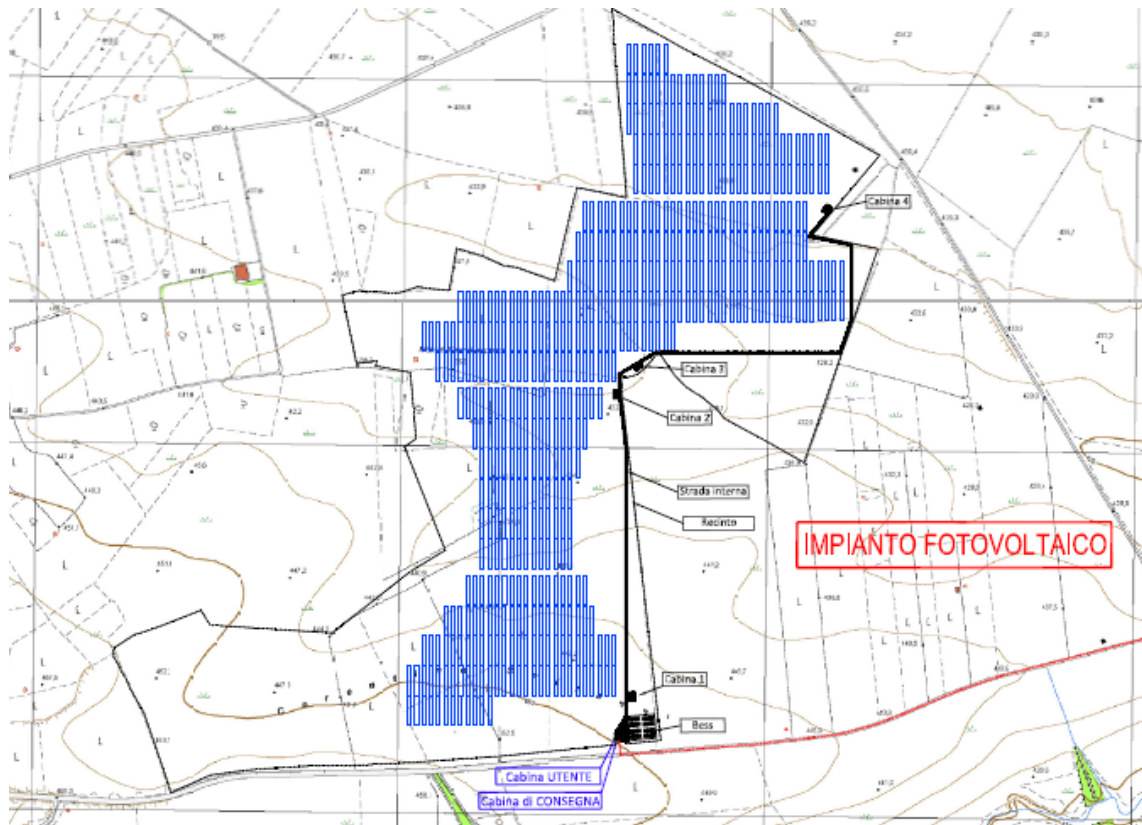
Figura 4 – Planimetria generale del sito di intervento
