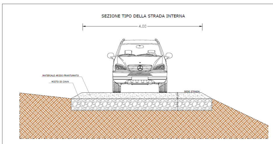
Figura 17 sezione tipo strada interna
