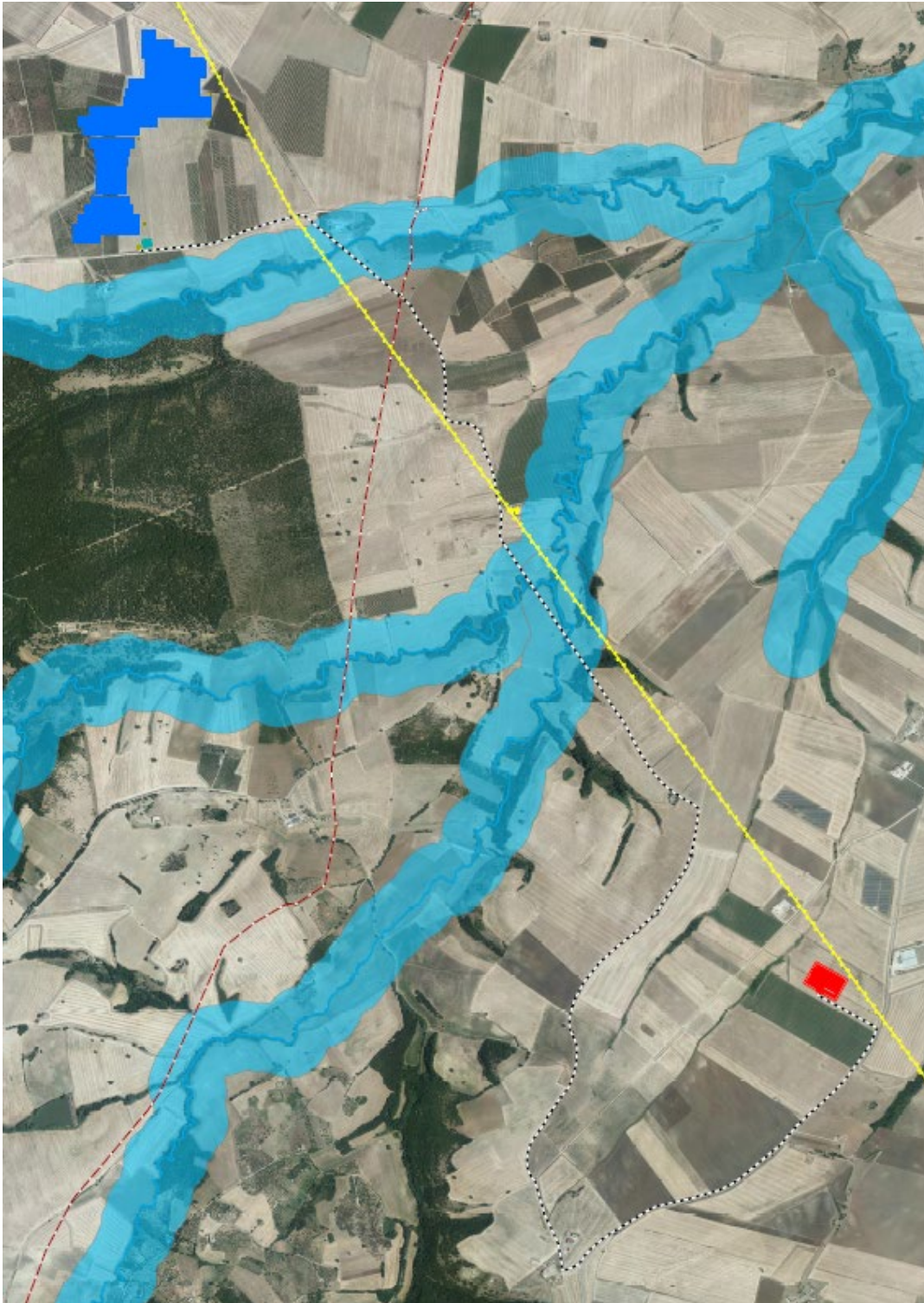
Figura 12 – Carta delle interferenze
