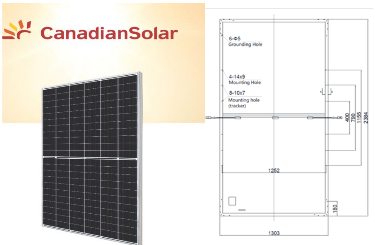
Figura 11 – Modulo fotovoltaico
