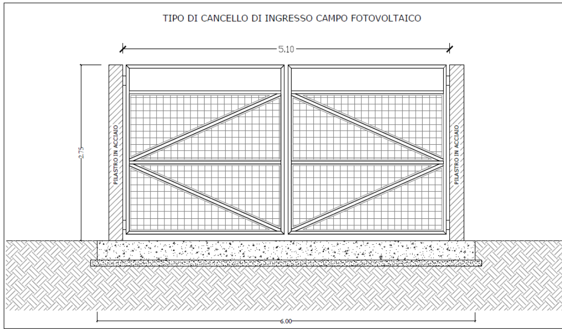
Figura 23 - Cannello di ingresso al campo fotovoltaico
