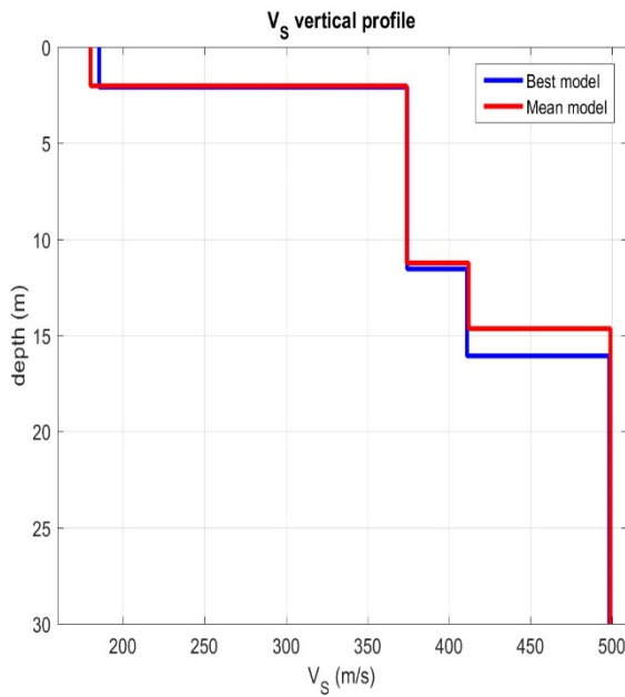
Figura 5-Profilo V_{S, equ} = 357 m/sec calcolato a partire dal piano campagna
