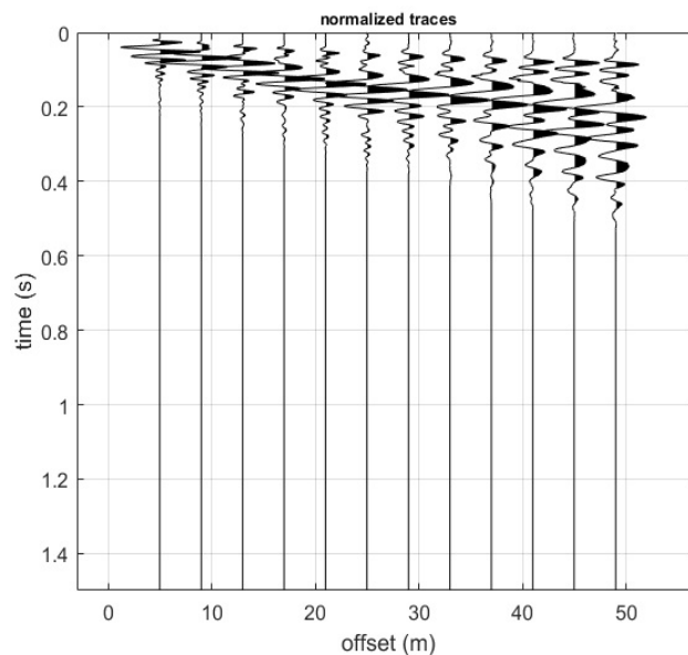
Figura 9-Tracce acquisite in situ ed utilizzate per la costruzione dello spettro di
