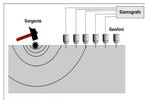
Figura 2-Schema realizzativo indagine MASW (Onde di
