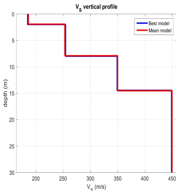
Figura 11-Profilo V_{S, equ} = 343 m/sec calcolato a partire dal piano campagna
