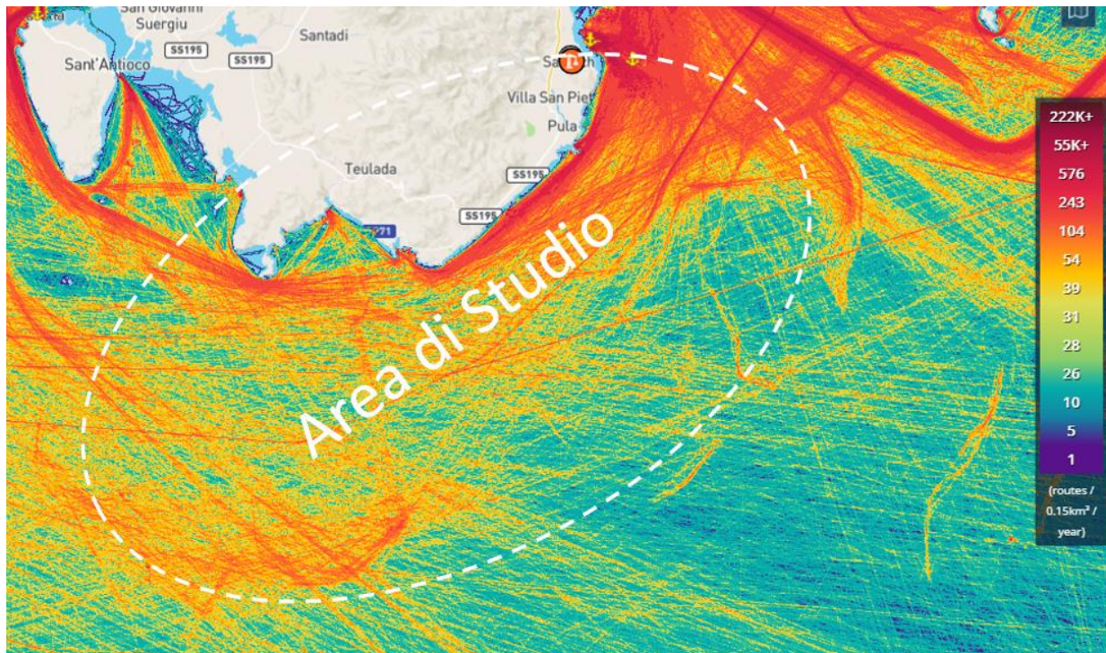
Figura 4.2: Mappa della Densità del Traffico Marittimo annuale di fronte alle coste dell'Area di Studio del 2019
