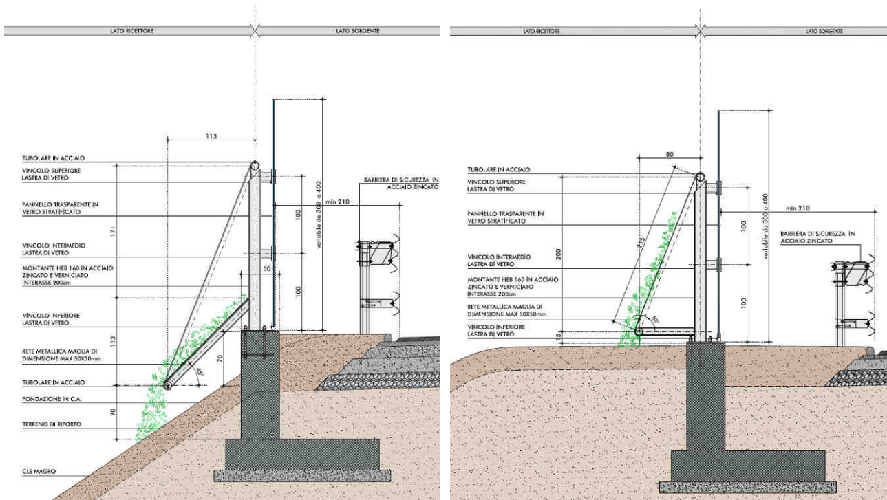
FIGURA 5-6 – SEZIONE TIPOLOGICA DELLA BARRIERA ACUSTICA FONOSOLANTE TRASPARENTE TIPO 1 SU RILEVATO (SINISTRA) E PRESSO ALLARGAMENTO RILEVATO (DESTRA)
