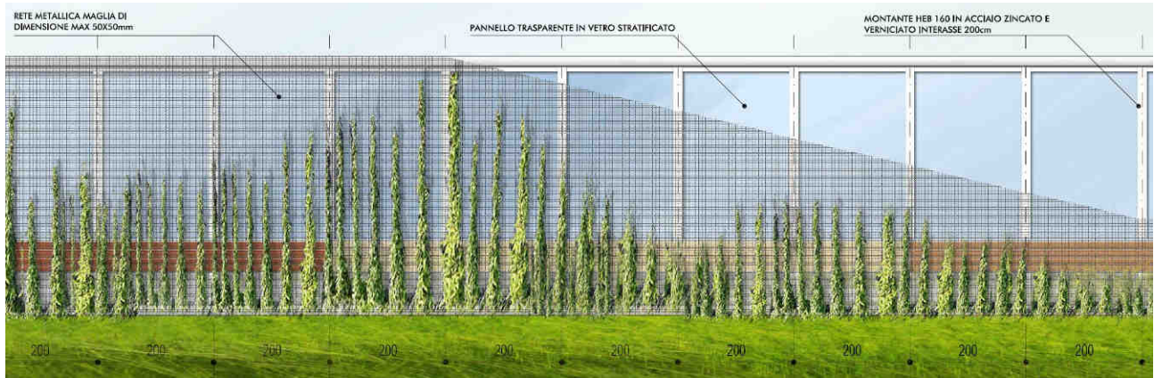
FIGURA 5-10 – BARRIERA ACUSTICA FONOIOLANTE TRASPARENTE TIPO 2 – PROSPETTO LATO RICETTORE
