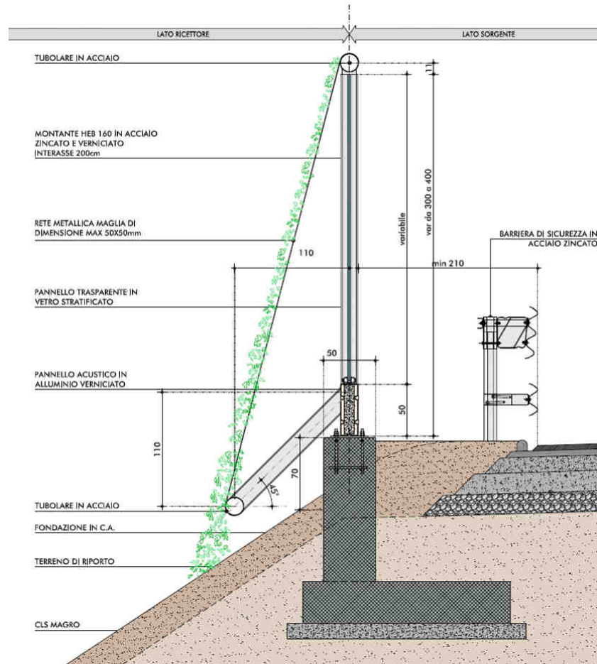
FIGURA 5-8 – BARRIERA ACUSTICA FONOIOLANTE TRASPARENTE TIPO 2 – SEZIONE TIPOLOGICA SU RILEVATO
