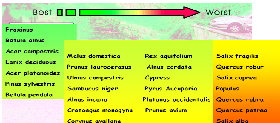
FIGURA 5-12 - GRADO DI PREFERENZA DI GENERI/SPECIE VEGETALI IN RELAZIONE ALLA CAPACITA' DI RIDUZIONE DI INQUINANTI ATMOSFERICI (FONTE: IBIMET BOLOGNA)
