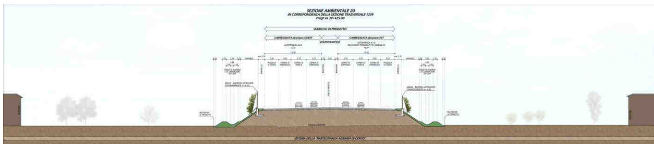
FIGURA 4-32 - SEZIONE SISTEMA DELLA "PARTECIPANZA AGRARIA DI CENTO"
