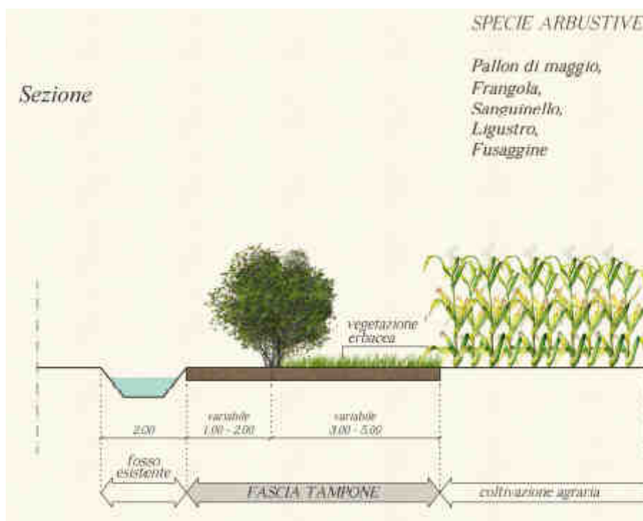
FIGURA 4-35 - ESEMPIO SEZIONE FASCE TAMPONE
