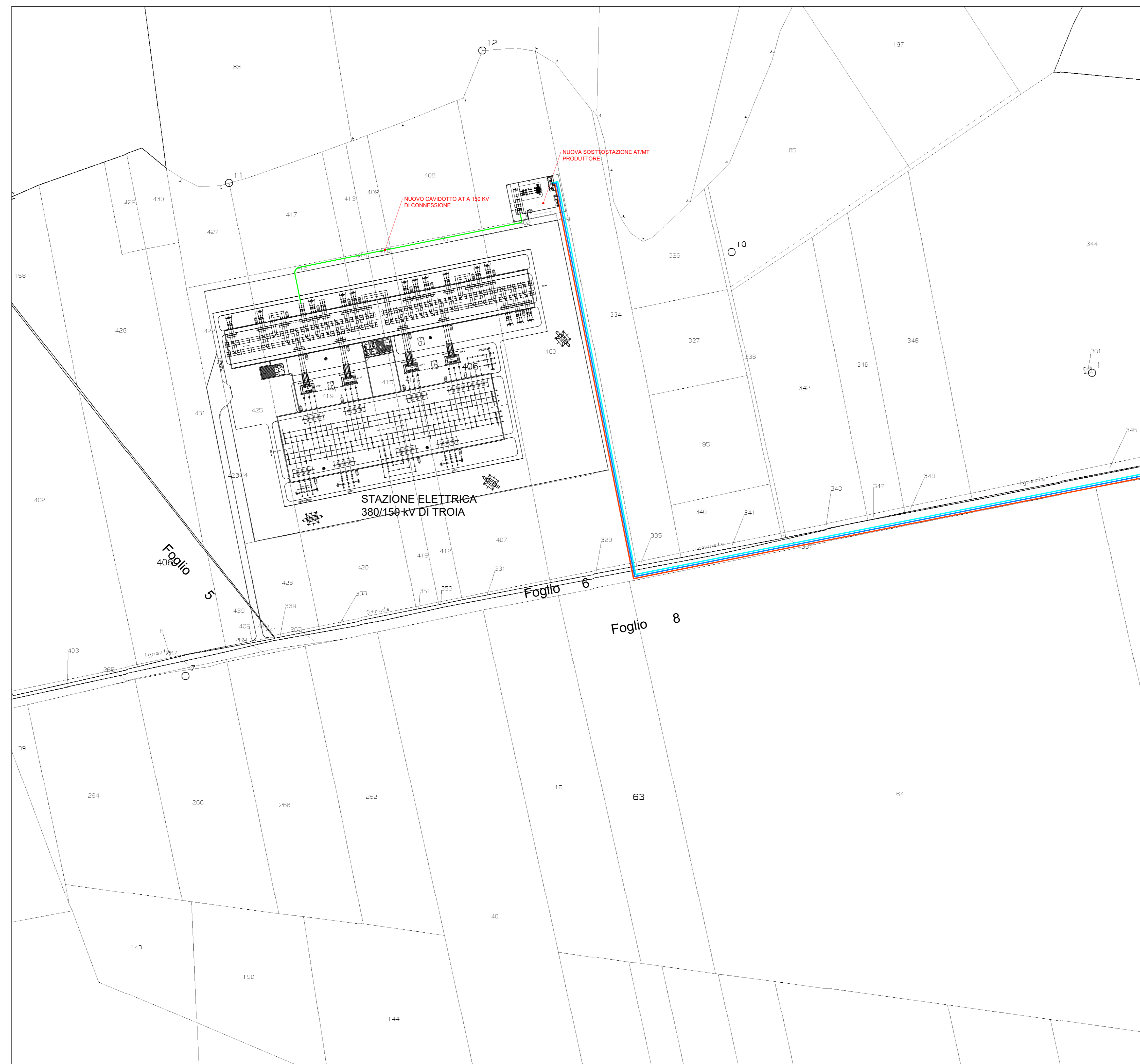
PLANIMETRIA OPERE DI CONNESSIONE UTENTE SU CATASTALE - SCALA 1:2000
