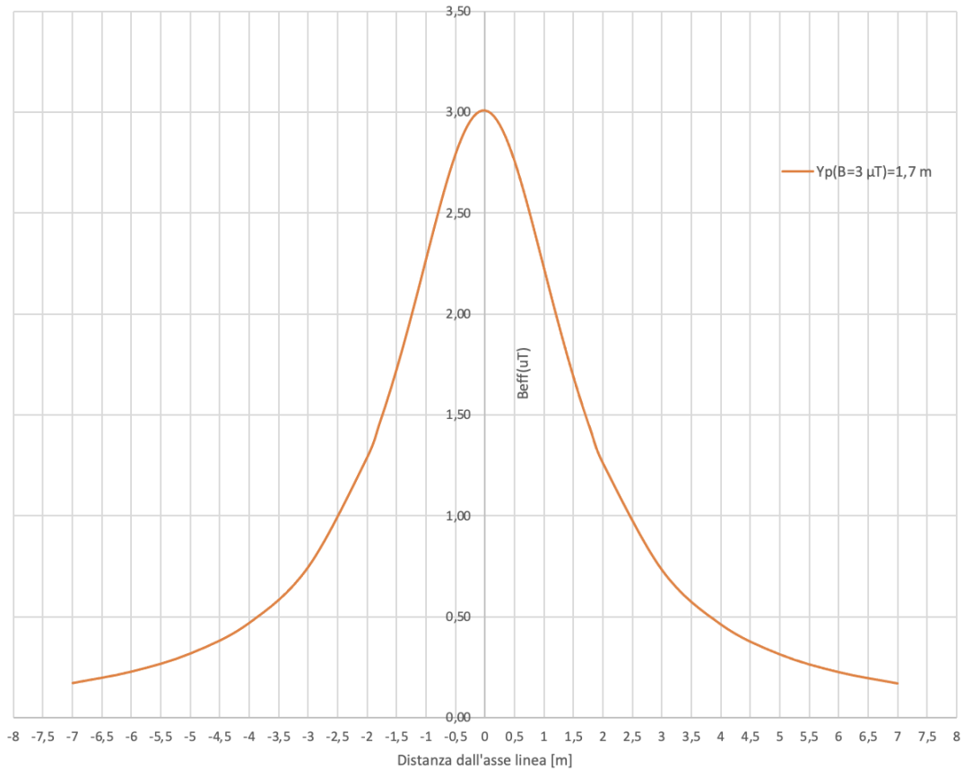
Figura 1: Profilo dell'induzione magnetica calcolata ad altezza Y_p(B=3 \mu T)=1,7 m di altezza dal suolo. Sezione cavo 630 mm 2 , corrente nominale 508 A.
