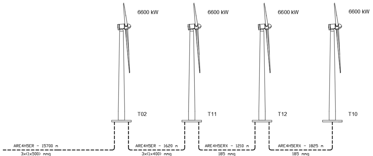
Schema a blocchi del parco eolico GRUPPO 3
