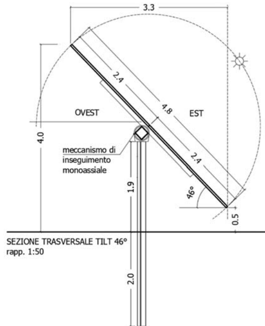
Sezione del tracker con inclinazione massima \pm 46^\circ - Disegno fuori scala
