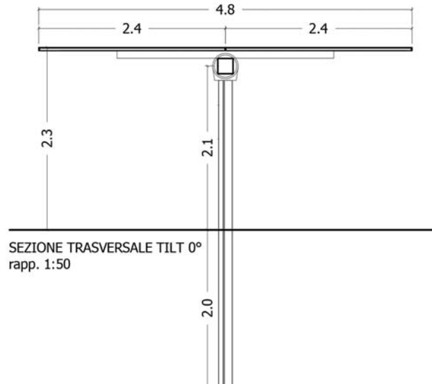
Tipico della struttura di supporto nella condizione di inclinazione 0^\circ – Disegno fuori scala
