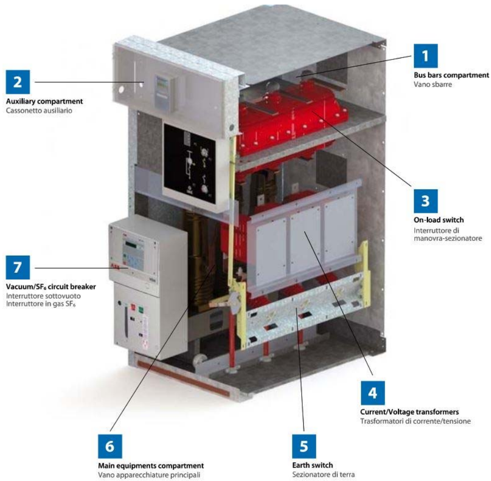
Esploso di uno scomparto MT tipico.
