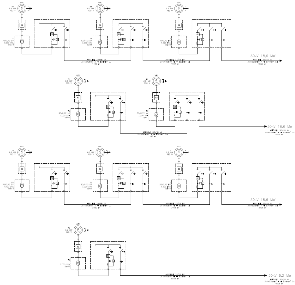
Figura 1: schema a blocchi parco eolico (circuiti 1, 2, 3 e 4)
