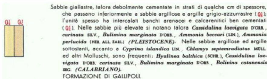
Stralcio del Foglio 203 della Carta Geologica D'Italia
