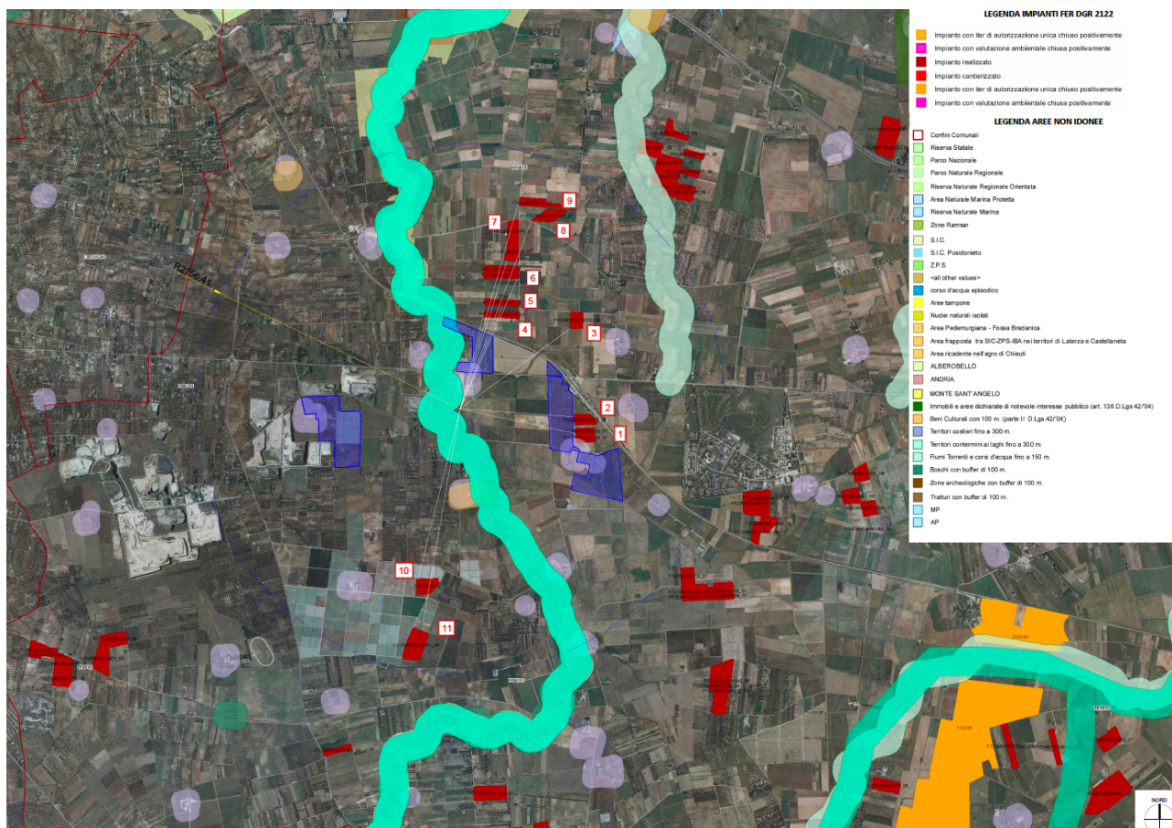
Tavola n. 1: Area vasta intorno all'impianto con r_{amb} = 2.756,51 m.
