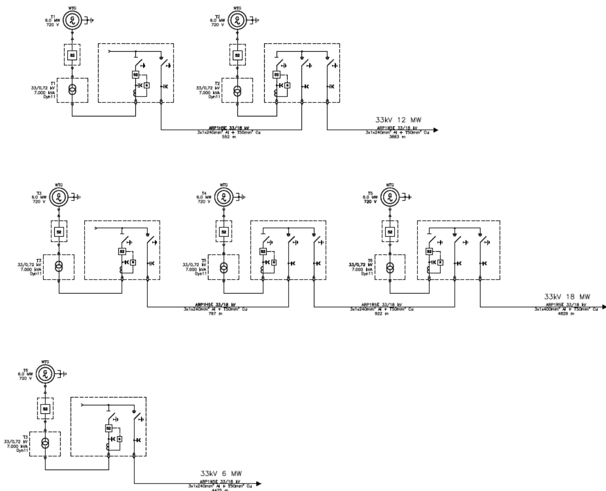
Figura 1: schema elettrico parco eolico
