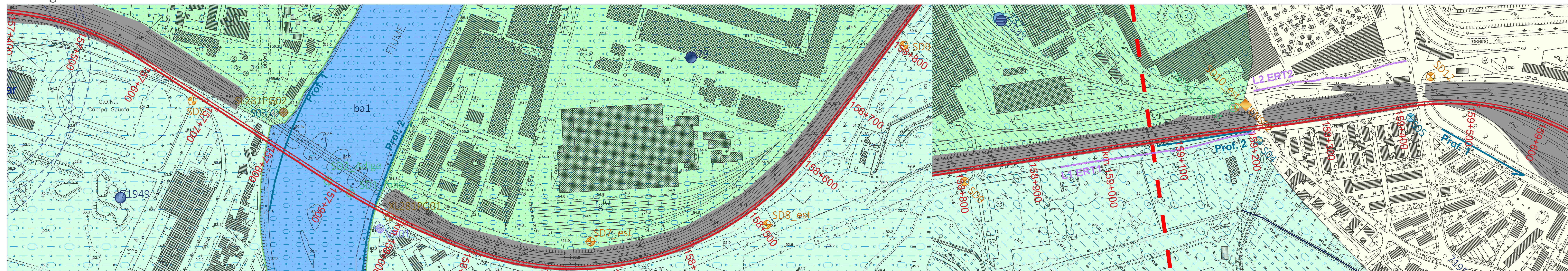
Profilo geologico Scala 1:2000/200
