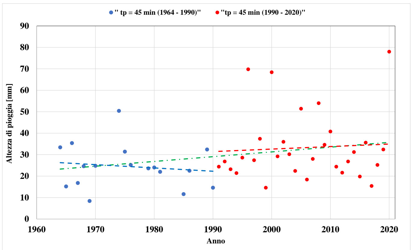
Figura 7: Altezze di pioggia massime annuali per tp=45 min, con linee di tendenza.
