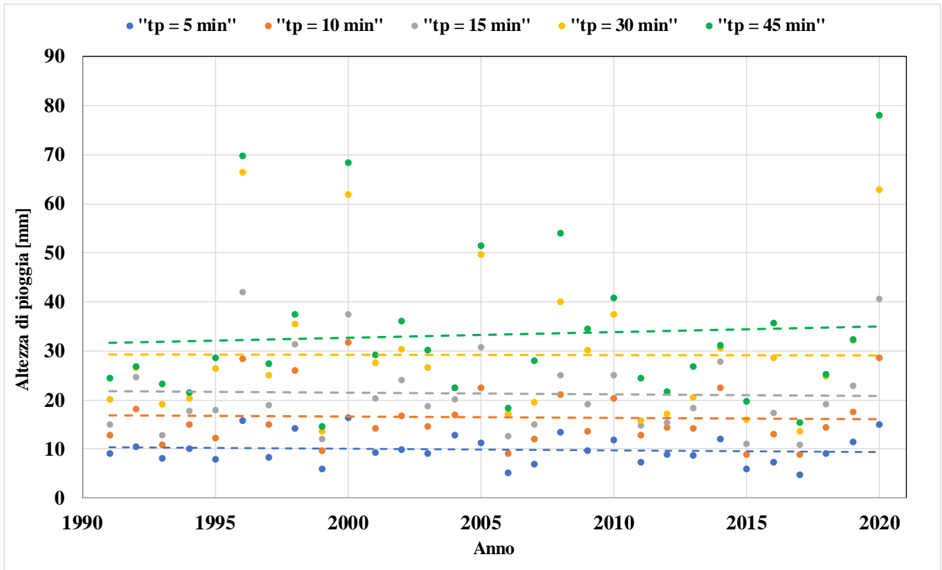
Figura 11: Grafico di comparazione delle linee di tendenza relative agli scrosci, periodo 1990-2020
