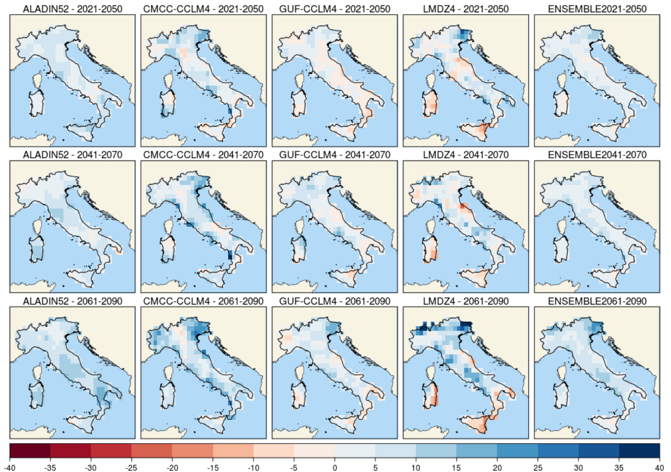
Figura 13 – Variazioni di precipitazione massima giornaliera (mm) previste dai modelli climatici per i tre orizzonti temporali 2021-2050, 2041-2070, 2061-2090, scenario RCP 8.5
