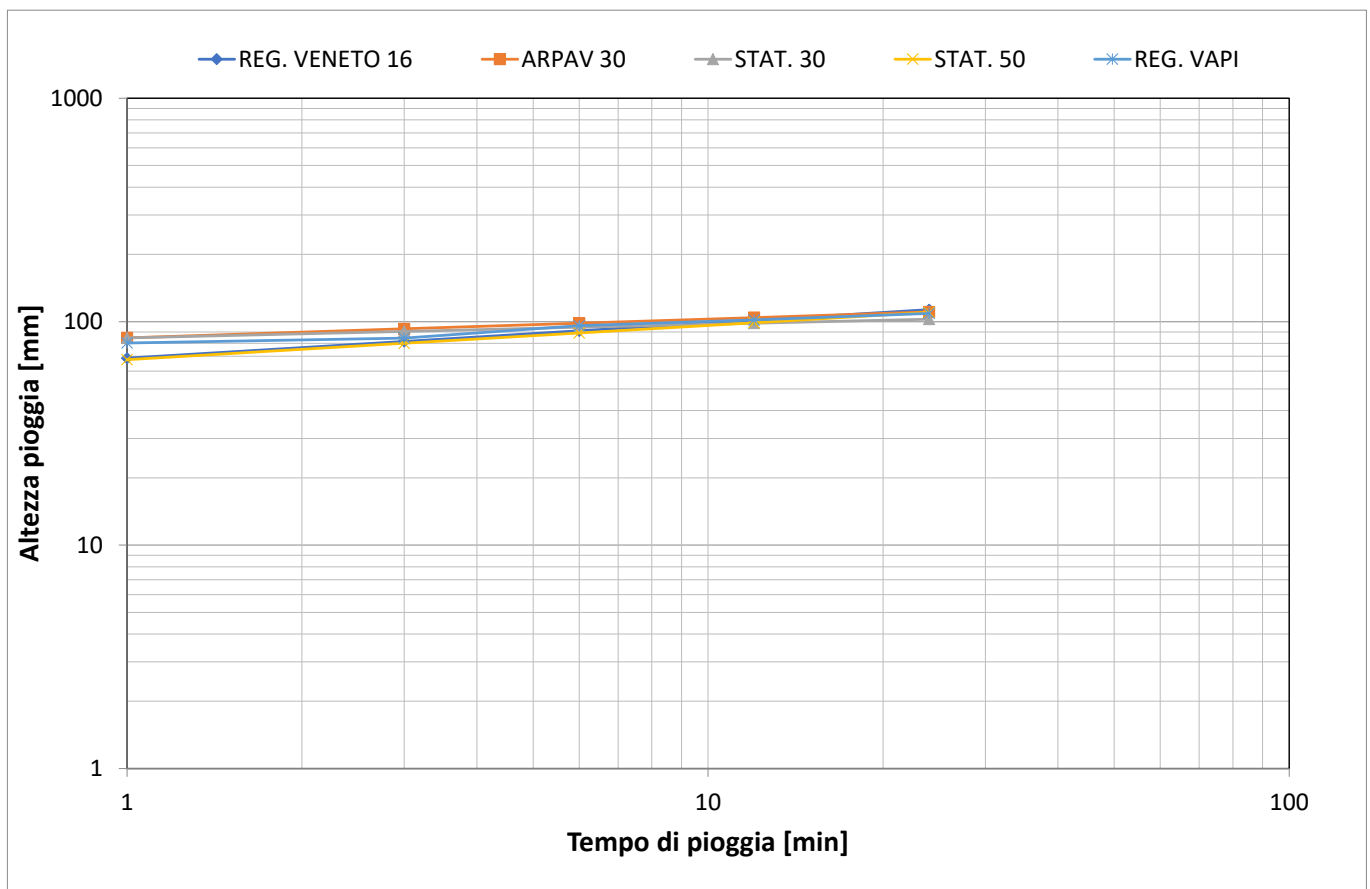
Figura 9: Valori di pioggia per durata precipitazione compresa tra 1h e 24h, Tr 50 anni
