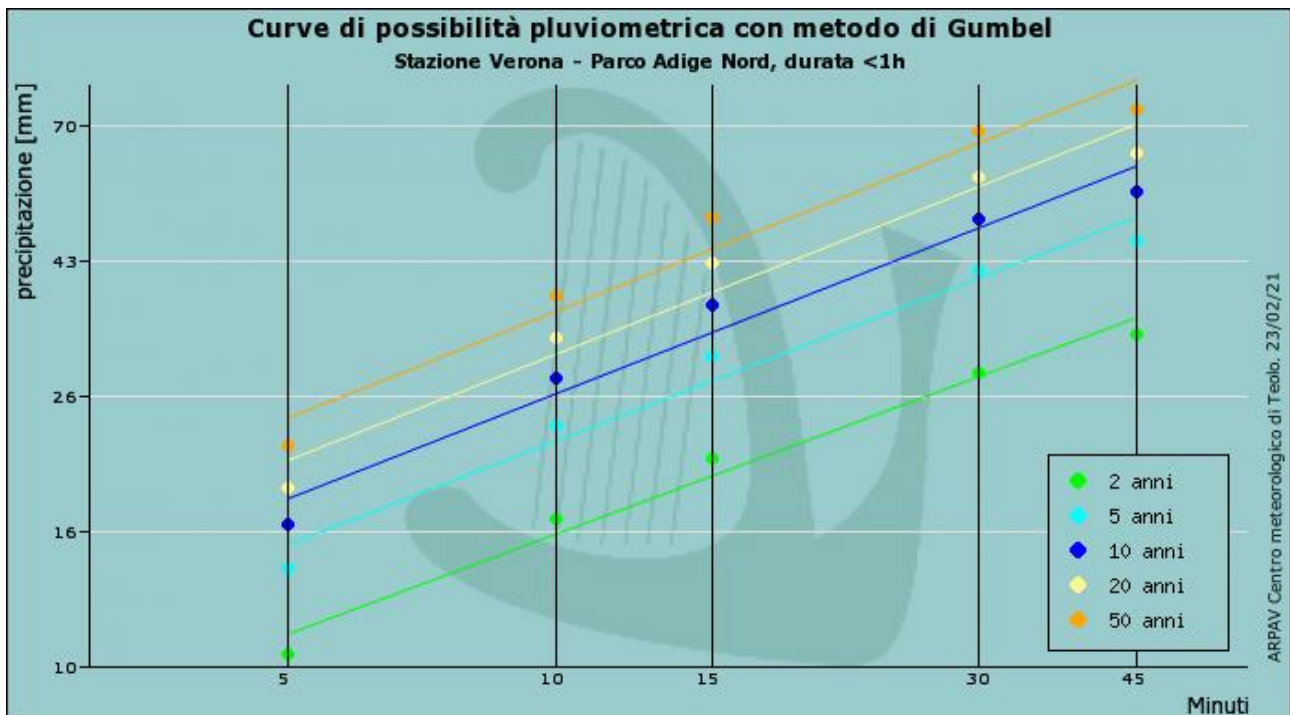
Figura 2: LSPP per durata precipitazione < 1h, Stazione Verona - Parco Adige Nord
