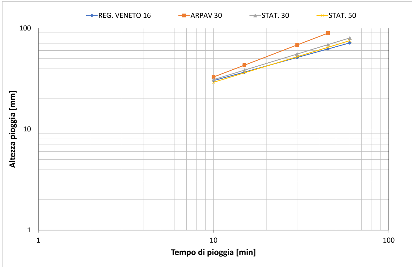
Figura 5: Valori di pioggia per durata precipitazione &lt; 1h, Tr 50 anni
