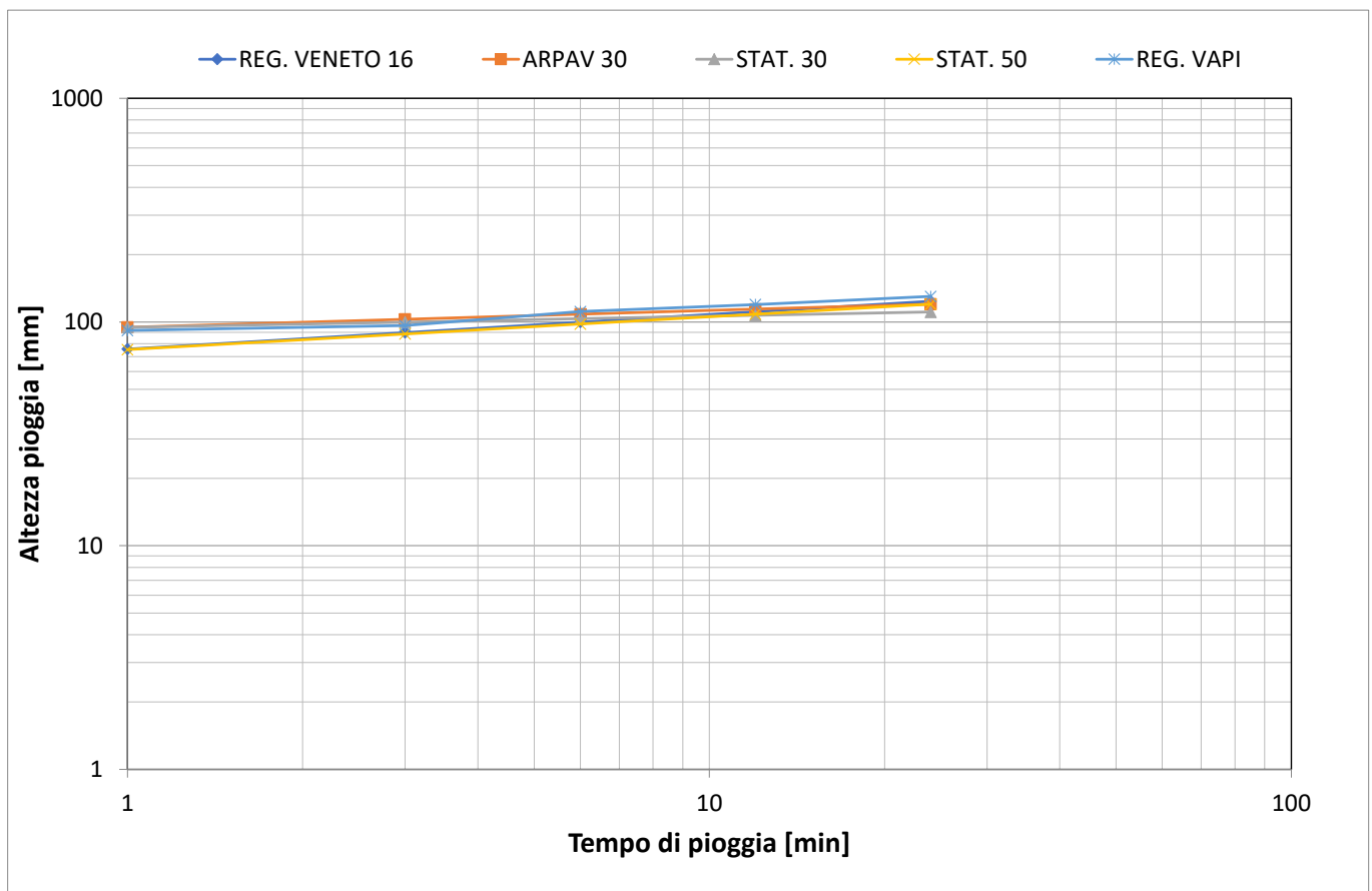
Figura 10: Valori di pioggia per durata precipitazione compresa tra 1h e 24h, Tr 100 anni
