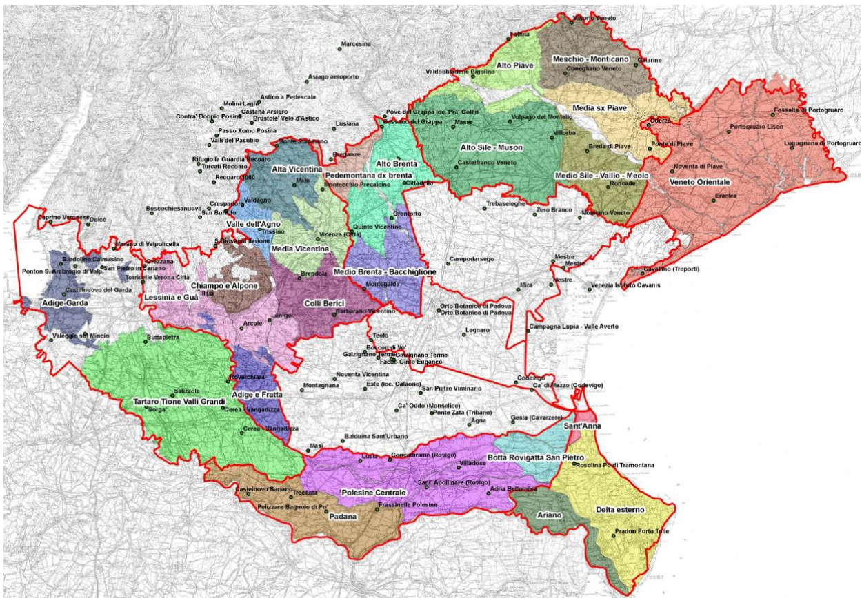
Figura 3: Delimitazione delle aree omogenee nell'Analisi regionalizzata della Regione Veneto.
