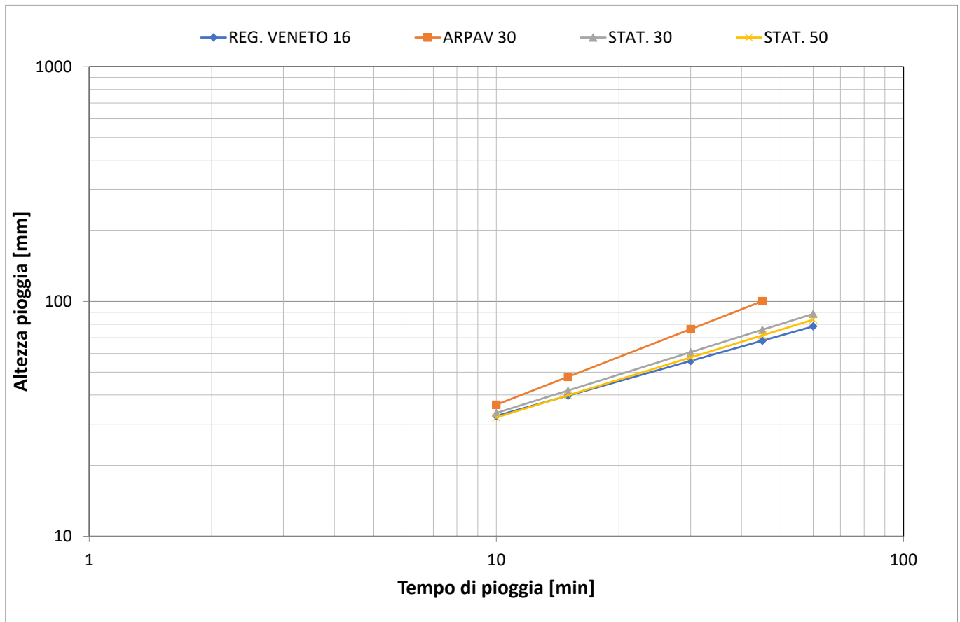
Figura 6: Valori di pioggia per durata precipitazione < 1h, Tr 100 anni
