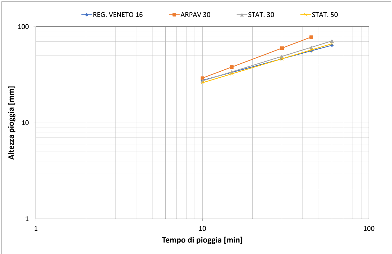
Figura 4: Valori di pioggia per durata precipitazione < 1h, Tr 25 anni
