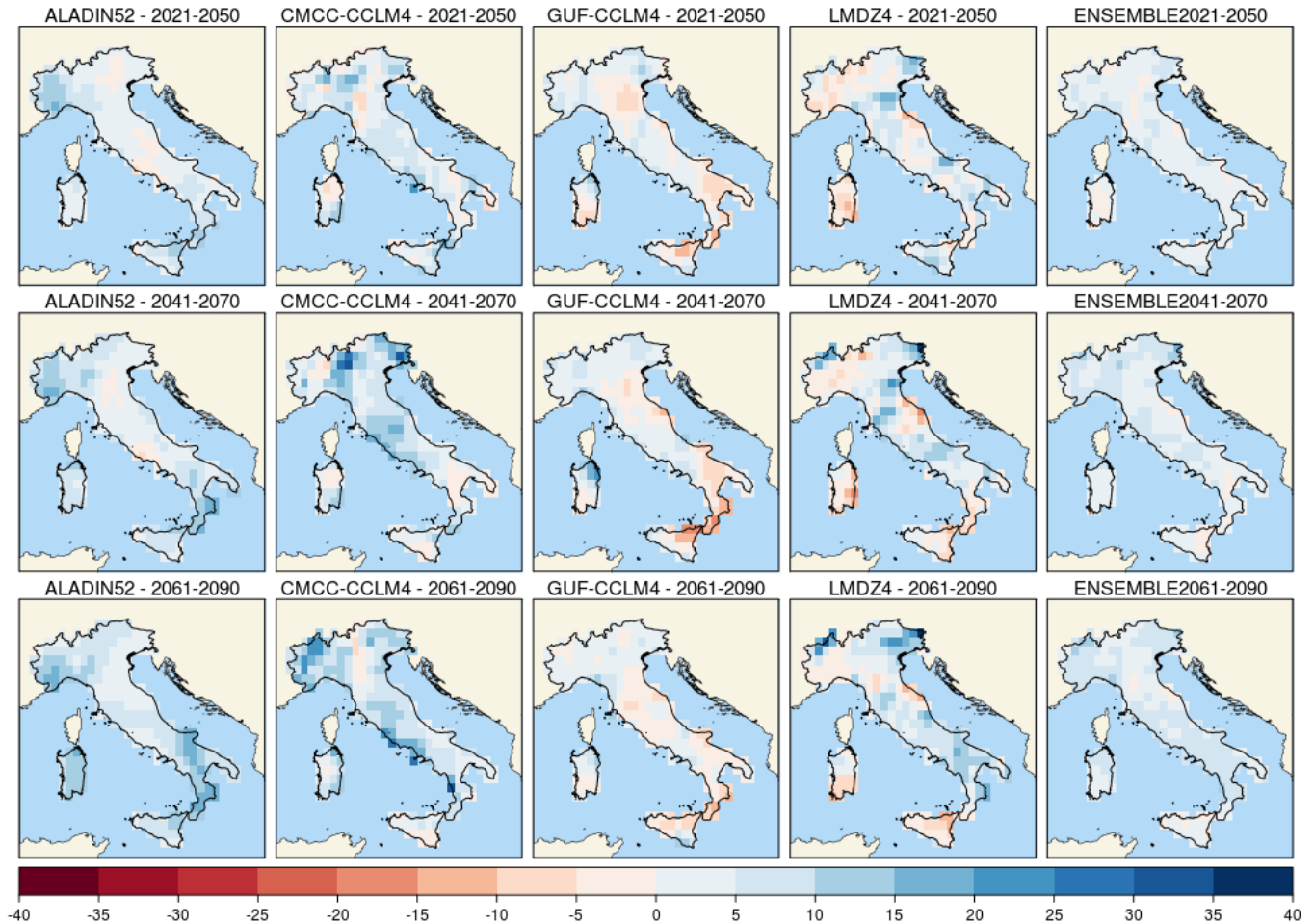
Figura 12 – Variazioni di precipitazione massima giornaliera (mm) previste dai modelli climatici per i tre orizzonti temporali 2021-2050, 2041-2070, 2061-2090, scenario RCP 4.5
