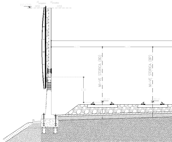
Figura - 9 Sezioni considerate per le verifiche
