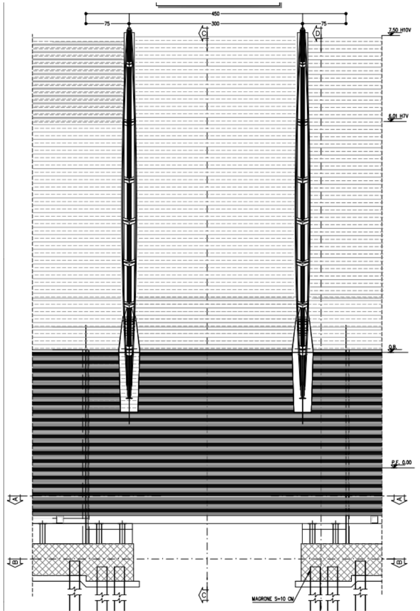
Figura - 2 Pianta e prospetto modulo di scavalco L=4.50m
