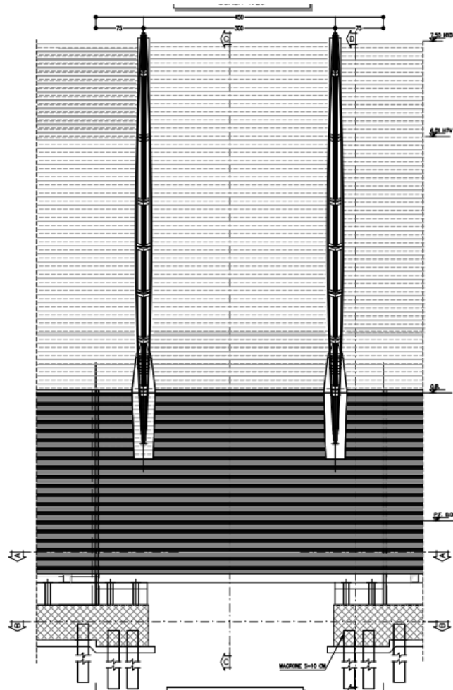
Figura - 1 Tipologico Scavalco L=4.50m
