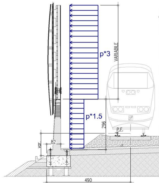
Figura - 6 Andamento della pressione del vento con l'altezza della barriera.
