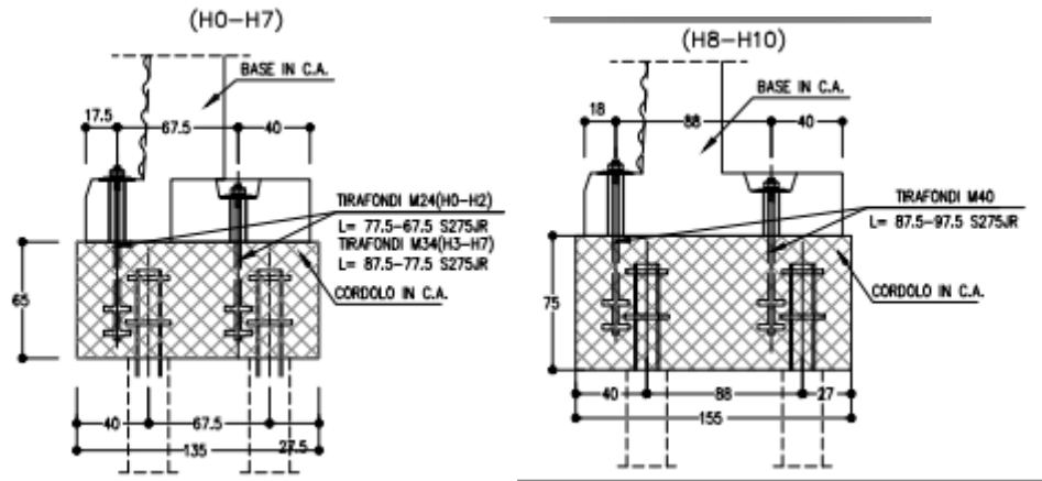
Figura - 3 Dettaglio fondazione
