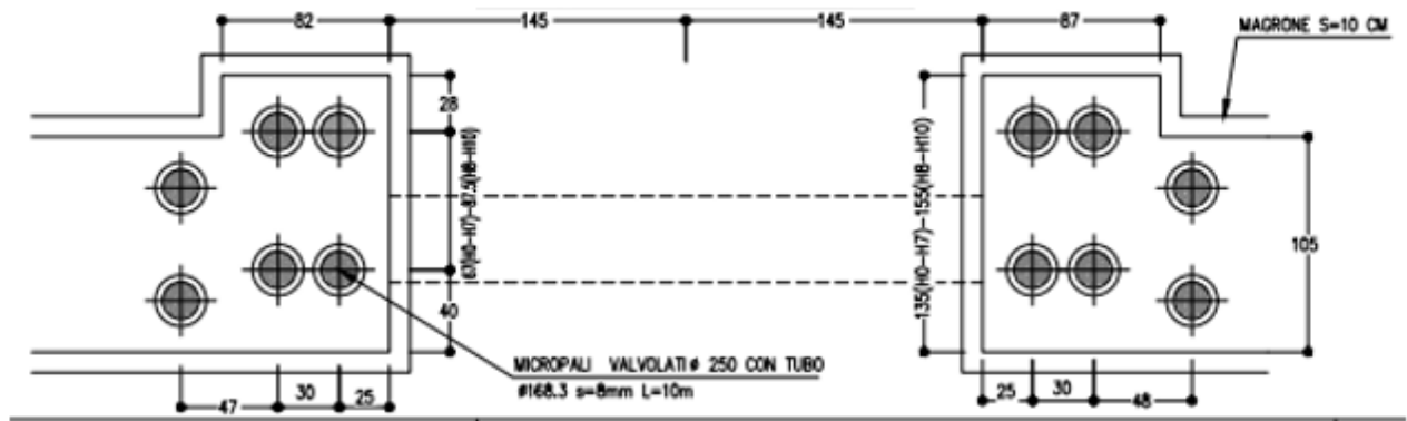
Figura - 4 Pianta fondazione
