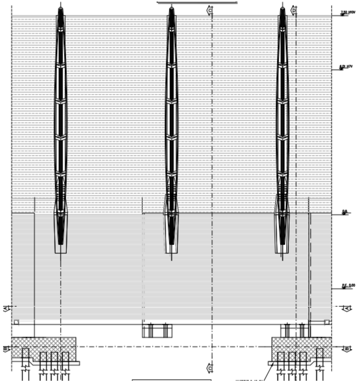
Figura - 1 Tipologico Scavalco L=7.50m
