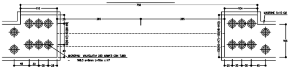
Figura - 3 Pianta fondazione
