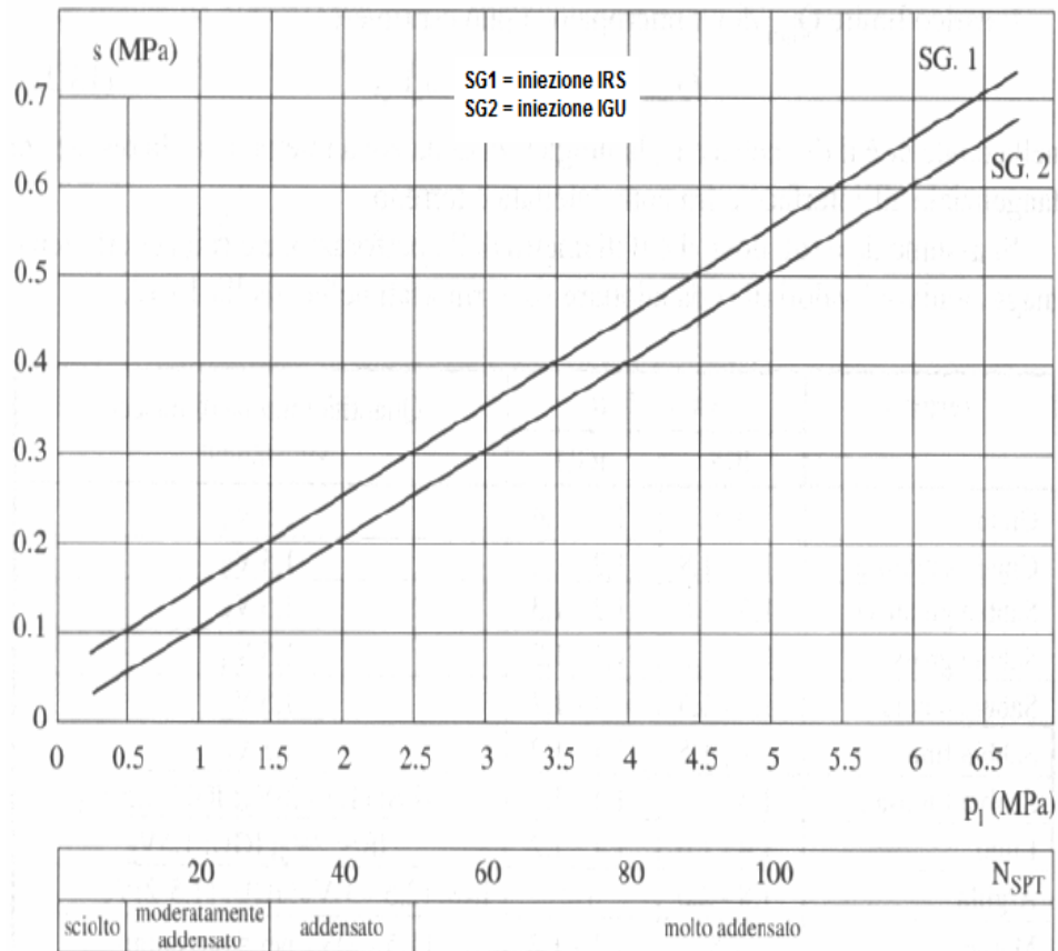
Figura - 9 Abaco per la determinazione di s per sabbie
