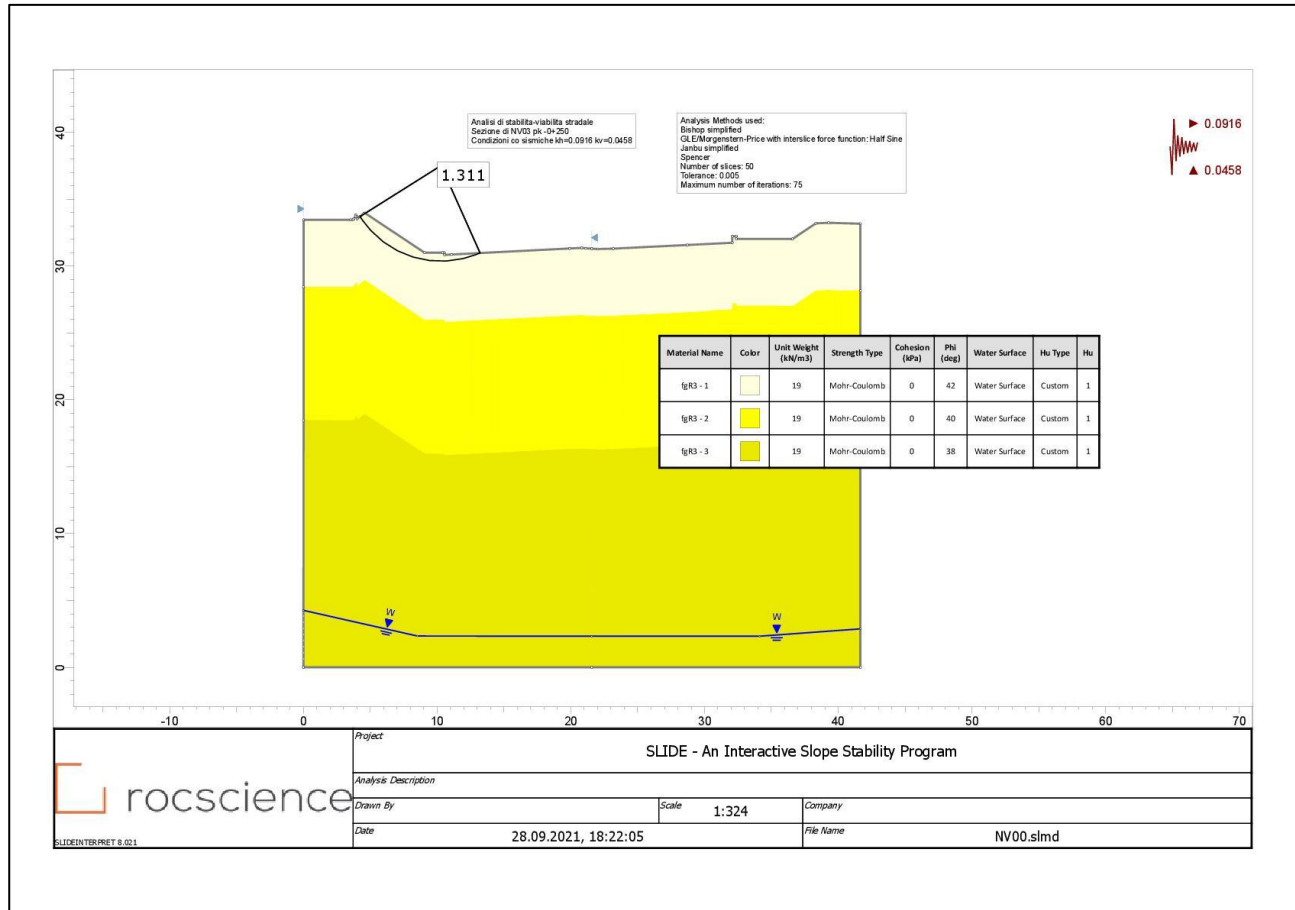
Figura 3: H=2.97 m, pk 0+250 di NV01 -Analisi di stabilità globale in campo sismico-condizioni co-sismiche (-)
