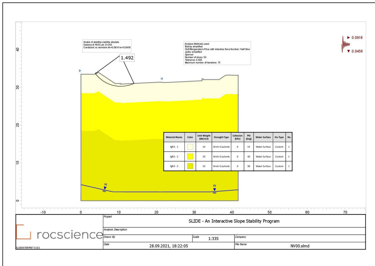
Figura 2: Trincea H=2.97 m, pk 0+250 di NV01 -Analisi di stabilità globale in campo sismico-condizioni co-sismiche (+)
