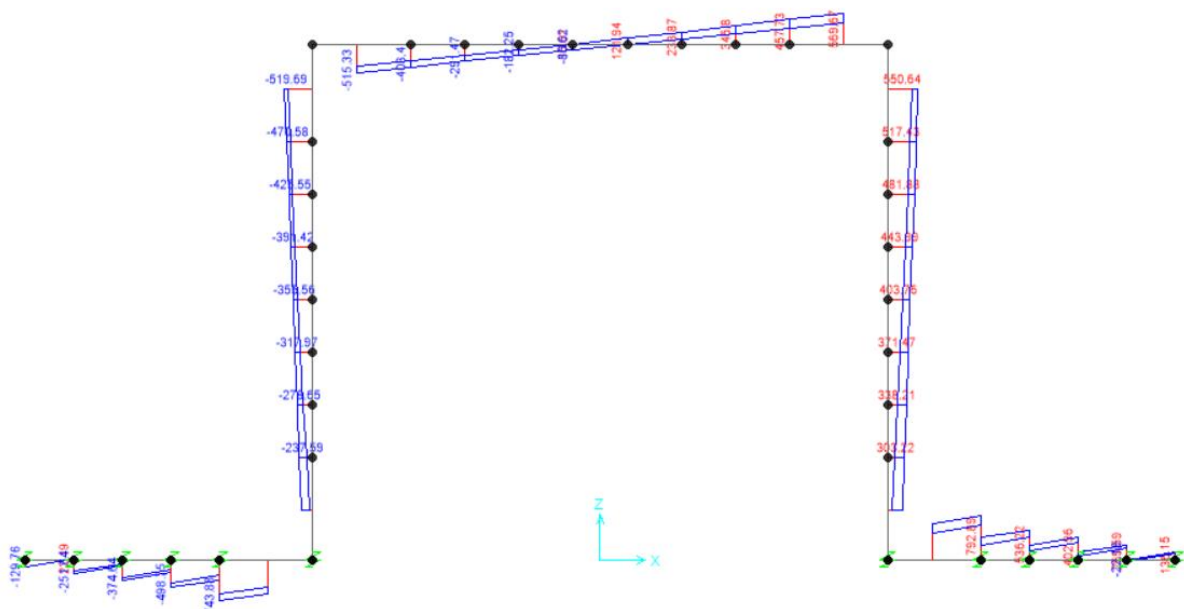
Fig. 5 – Involuppo sforzi taglienti SLU
