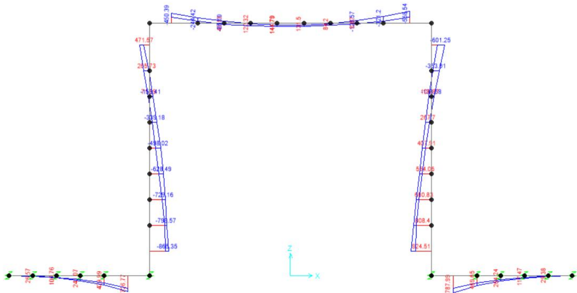
Fig. 4 – Involuppo momenti flettenti SLU
