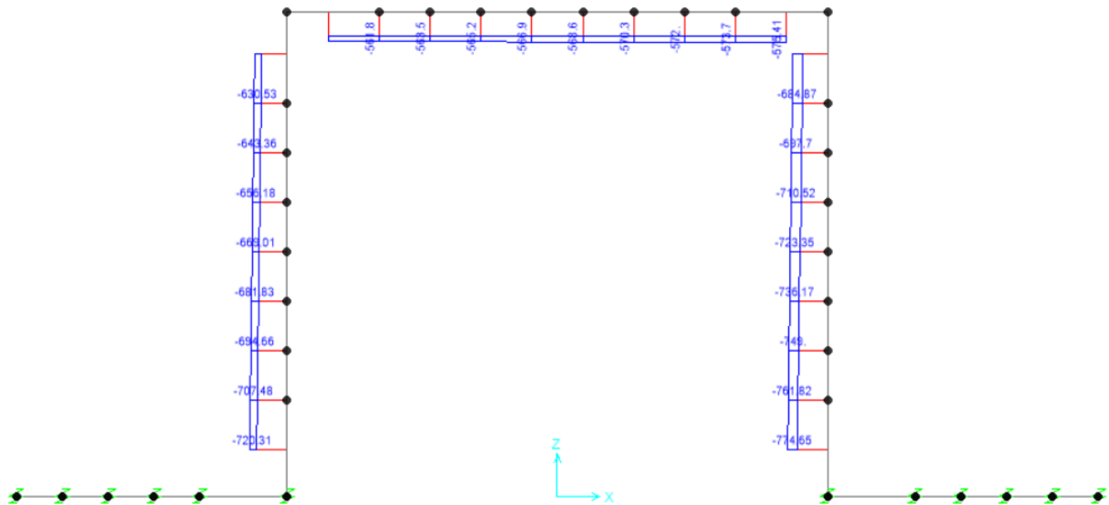
Fig. 6 – Involuppo azioni assiali SLU
