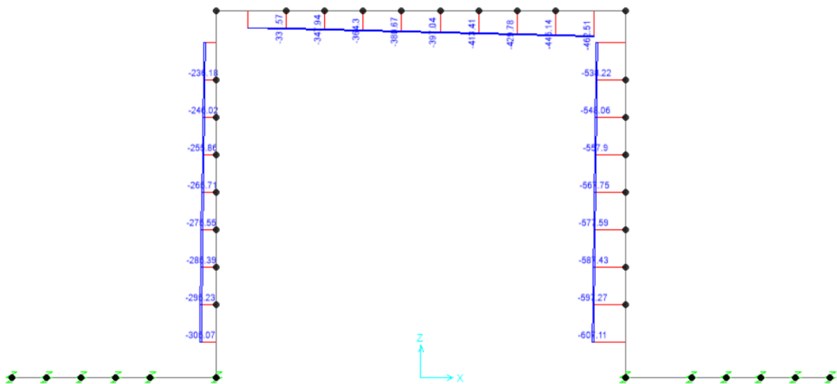
Fig. 9 – Involucro azioni assiali SLV
