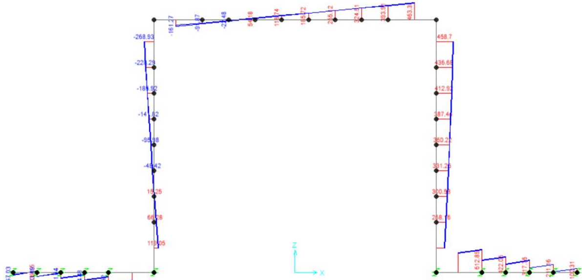
Fig. 8 – Involucro sforzi taglianti SLV
