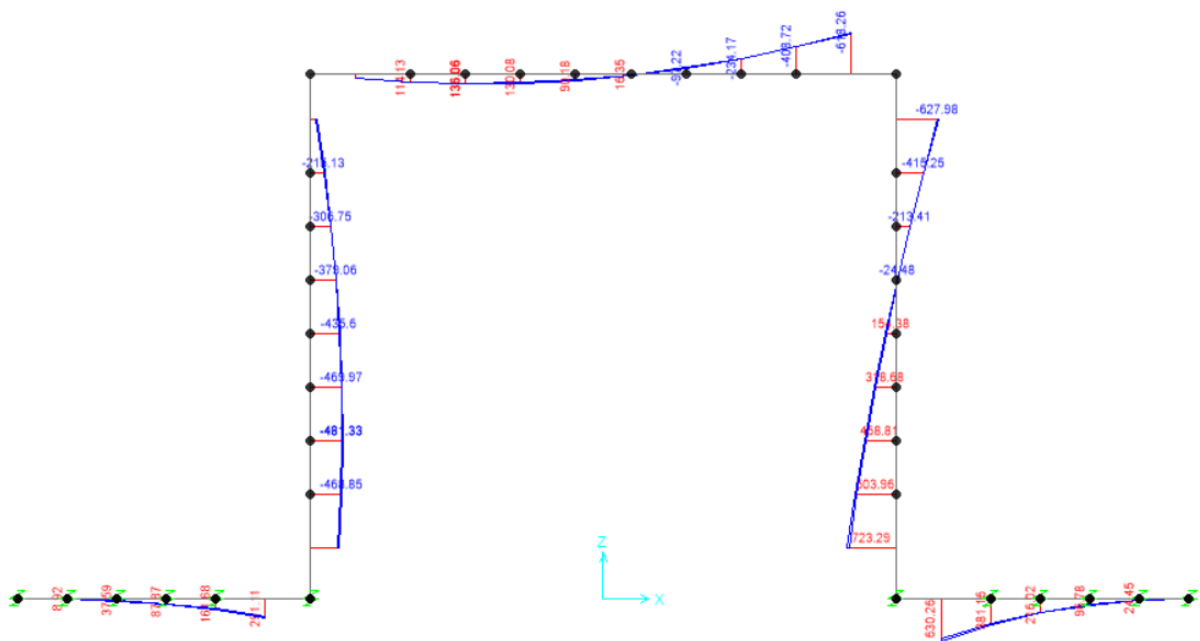
Fig. 7 –Involuppo momenti flettenti SLV
