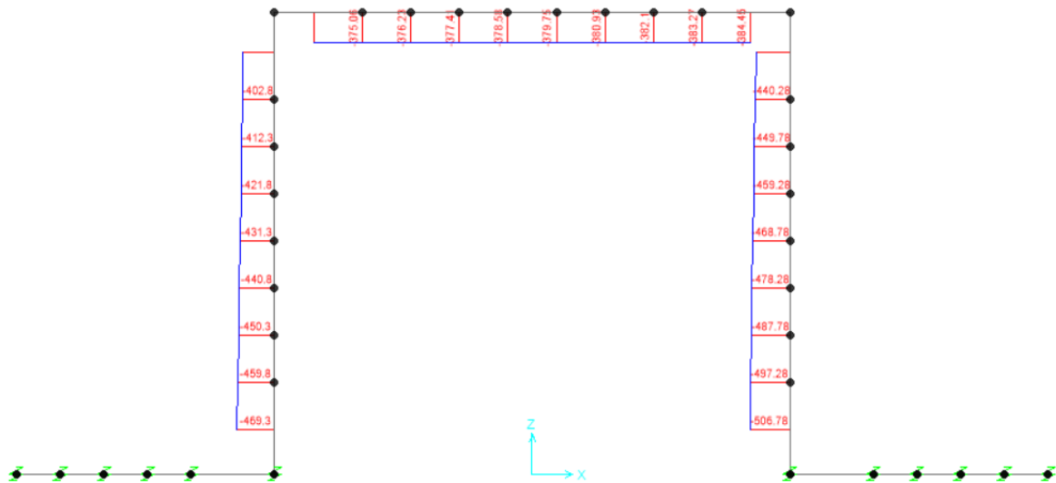
Fig. 11 – Involuppo azioni assiali SLE rara
