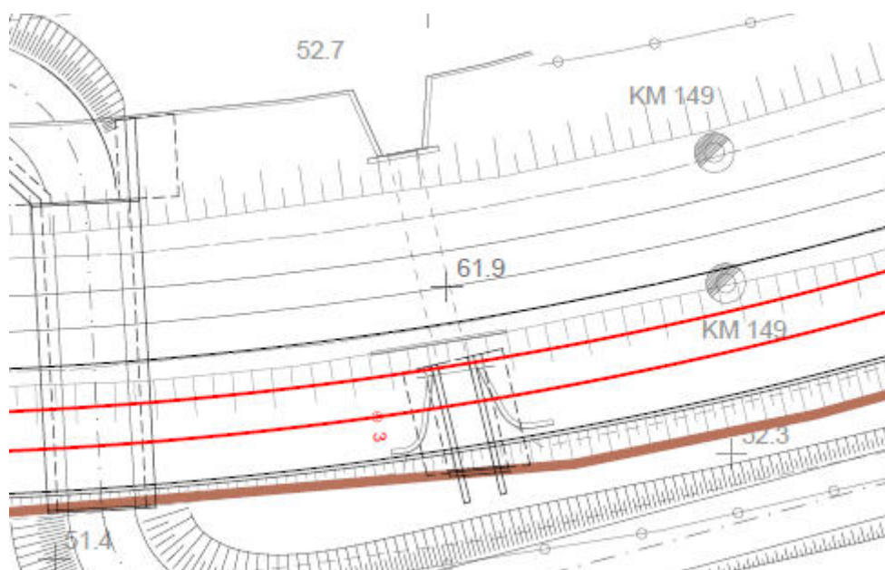
Figura 9 – Planimetria dell'intervento del sottovia ferroviario
