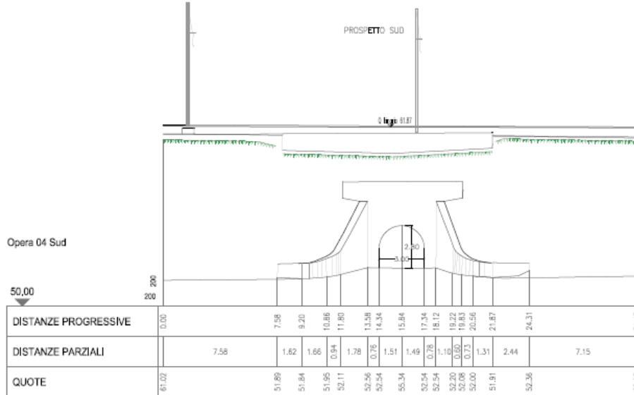
Figura 7 – Prospetto Sud
