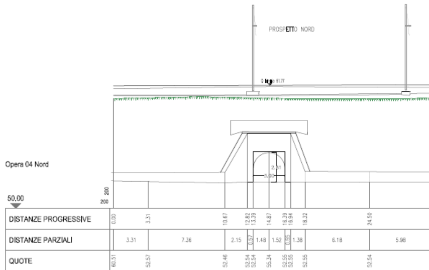
Figura 8 – Prospetto Nord
