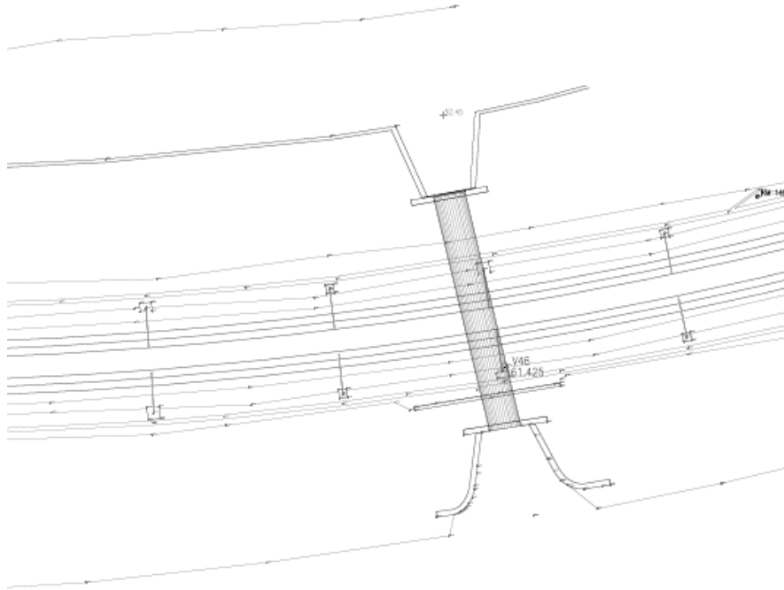
Figura 5 – Rilievo celerimetrico sottovia SL05
