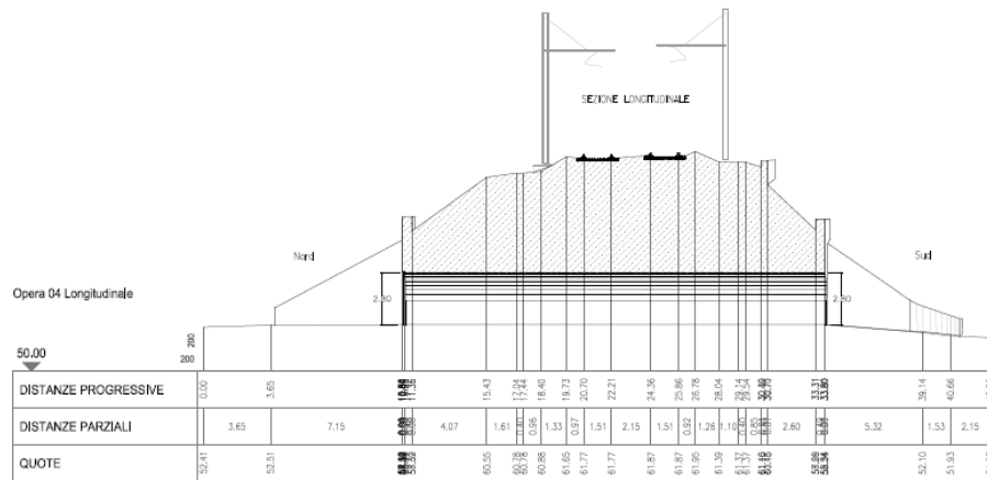
Figura 6 – Sezione longitudinale SL05
