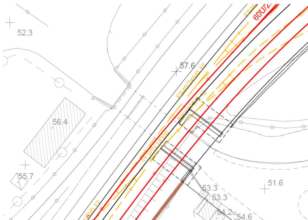
Figura 9 – Planimetria dell'intervento del sottovia ferroviario
