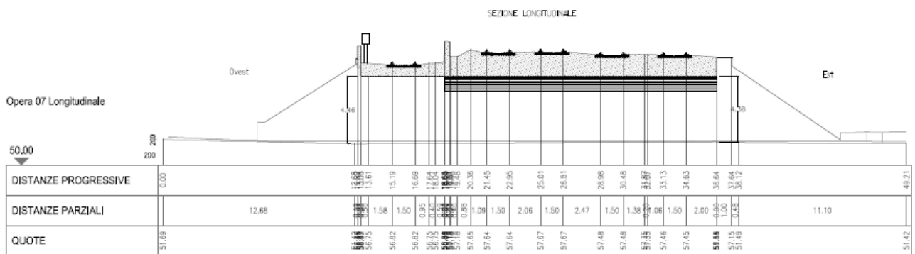
Figura 5 – Rilievo celerimetrico sottovia SL09
