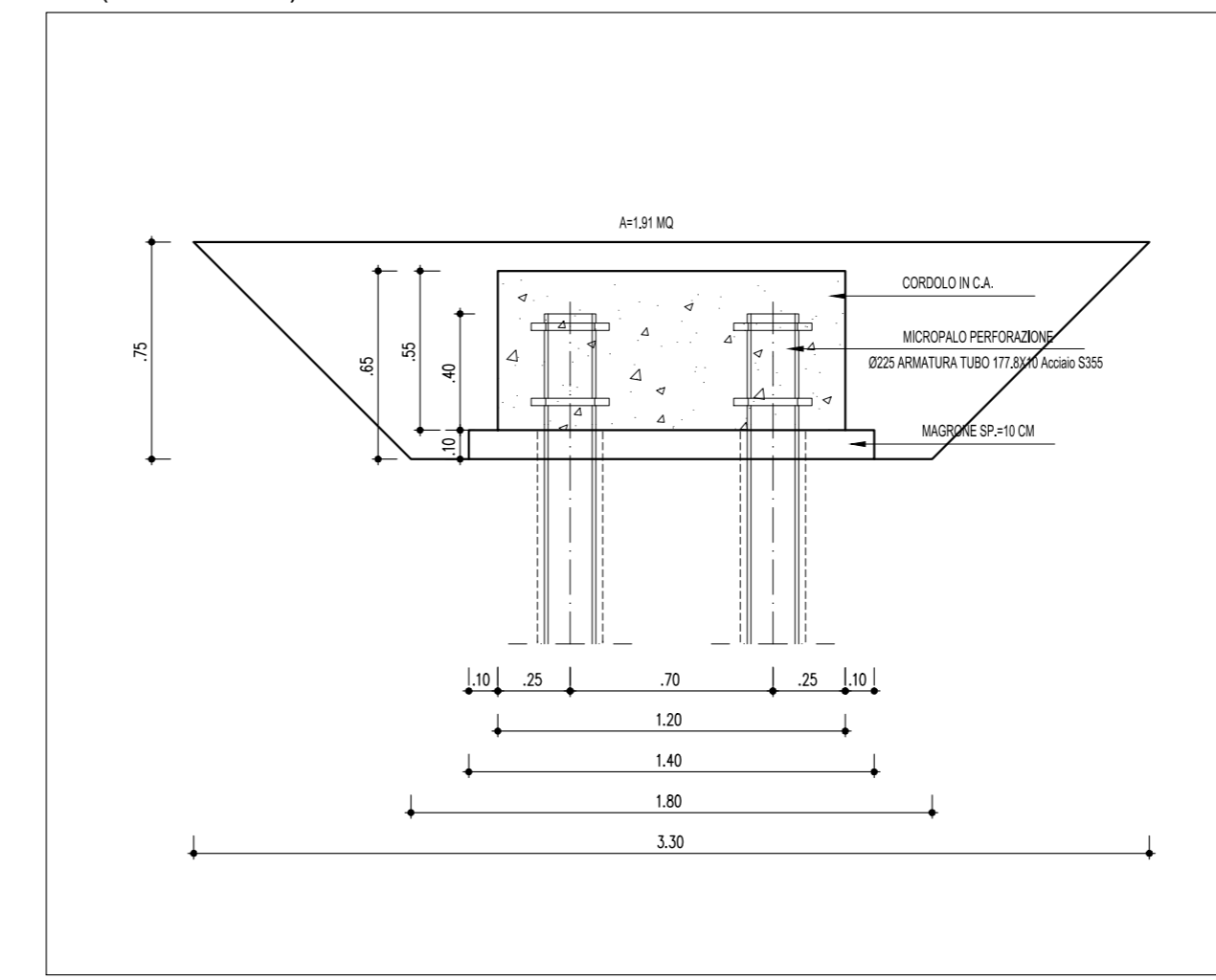
SEZIONE CORDOLO (SCALA 1:25)
