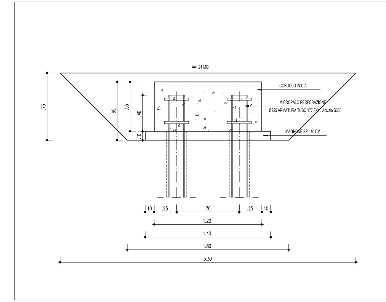
SEZIONE CORDOLO (SCALA 1:25)
