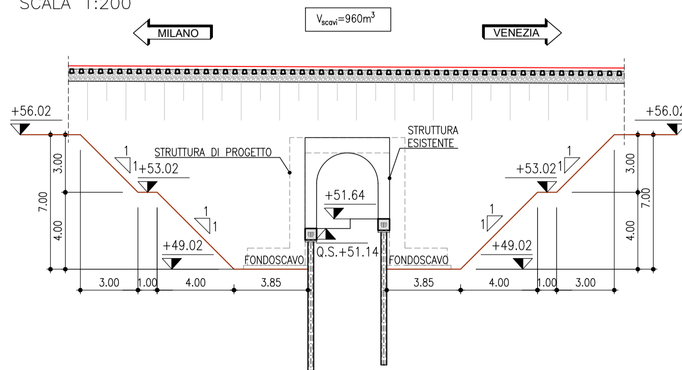
SEZIONE A-A SCALA 1:200
