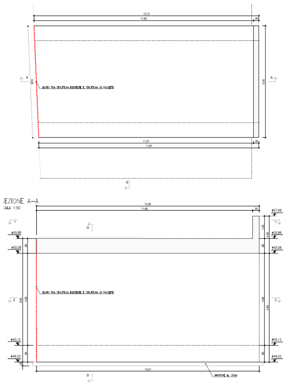
Figura 4 – Sezioni scatolare SL07
