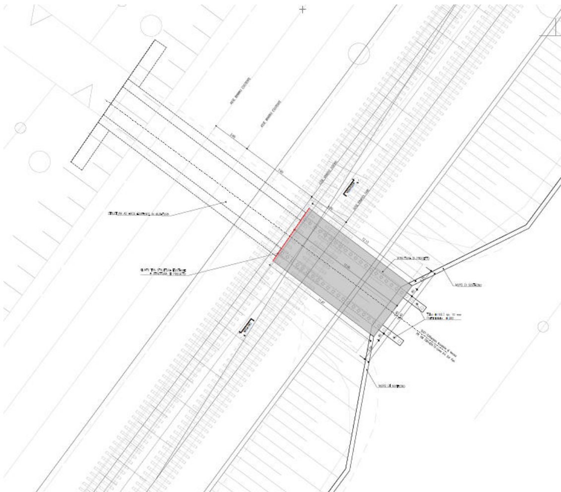
Figura 3 – Planimetria di progetto
