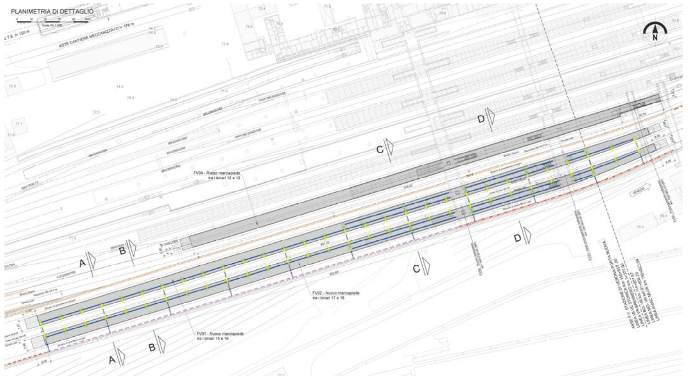
Figura 5: Stazione di Verona Porta Nuova - Marciapiedi
