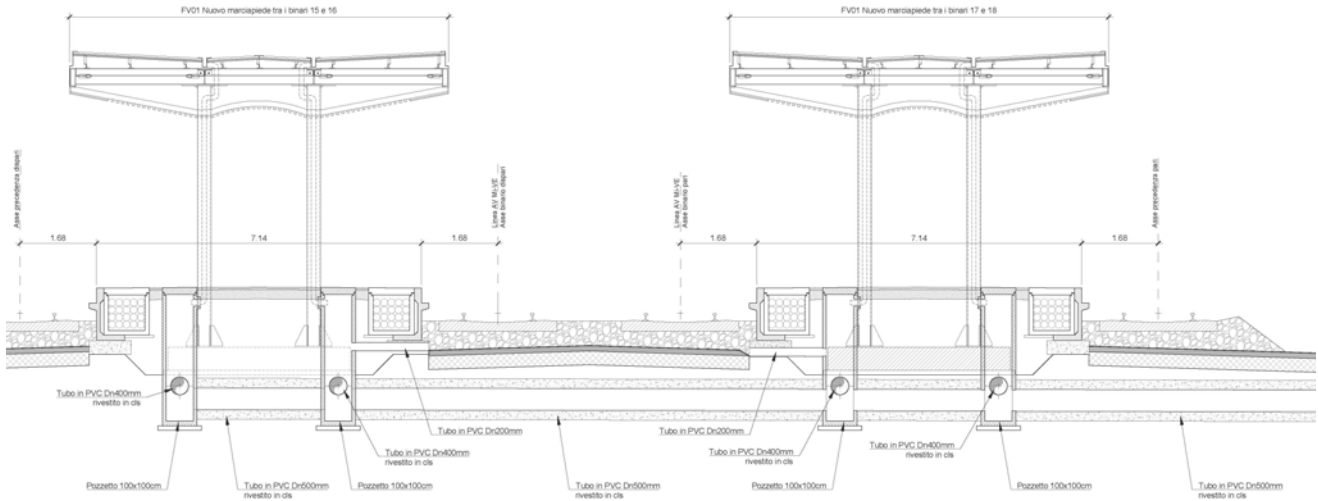
Figura 4: Stazione di Verona Porta Nuova - Collettori
