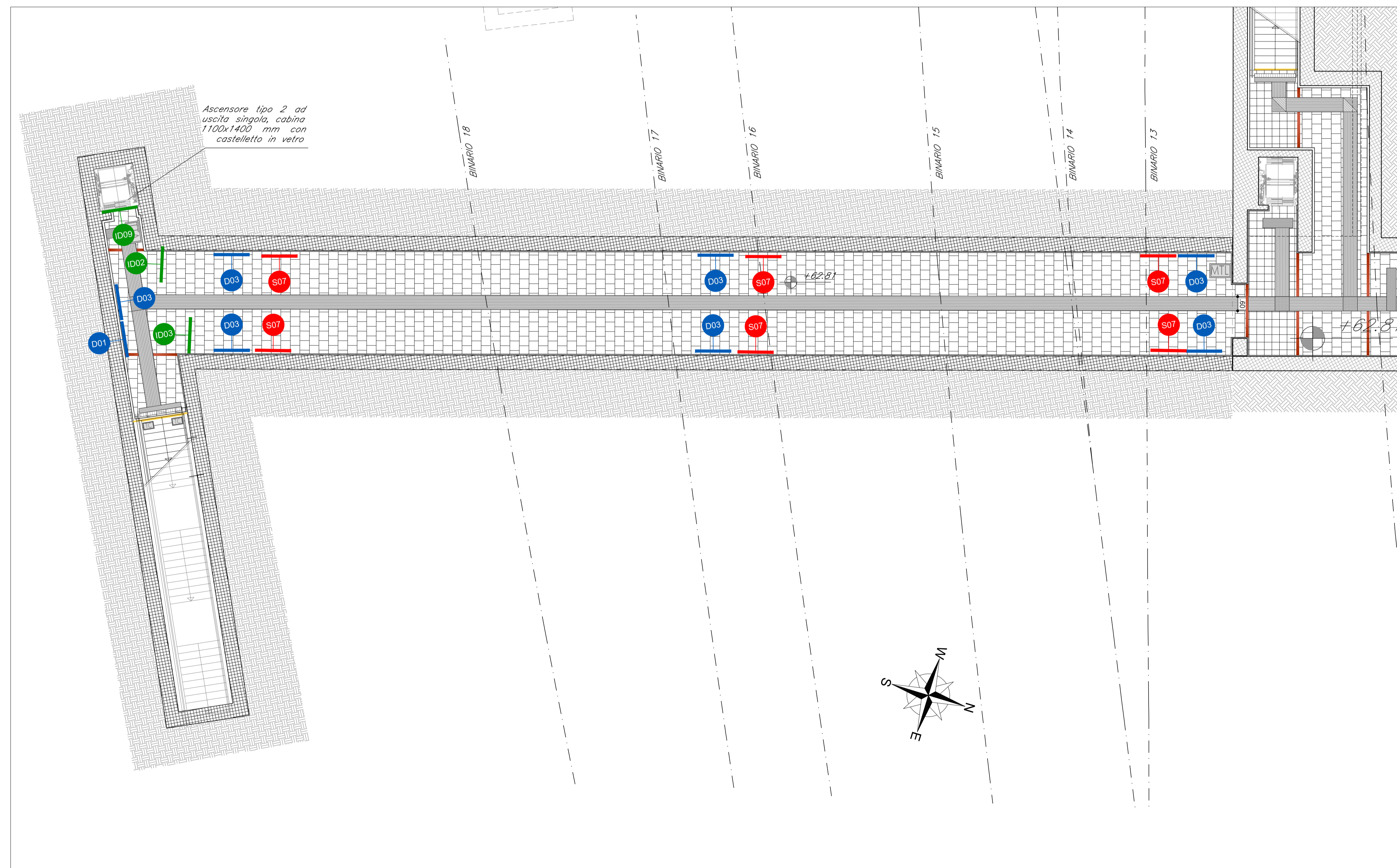
STRALCIO PLANIMETRICO PROLUNGAMENTO SOTTOPASSO scala 1:100
