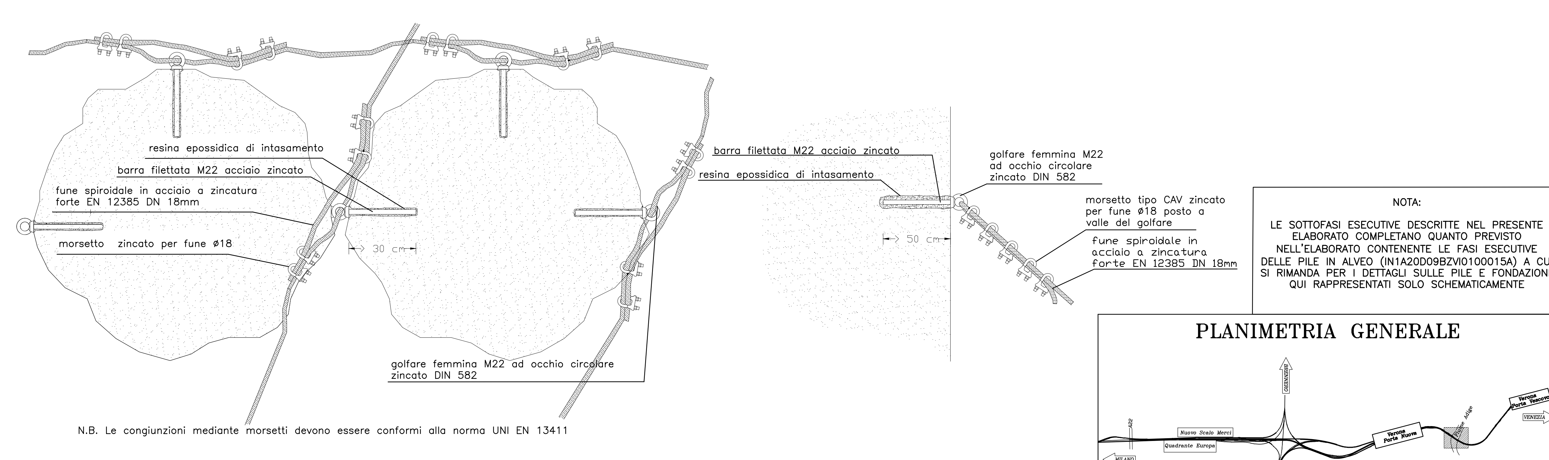
PARTICOLARE LEGATURA MASSI E AGGANCIAMENTO FUNE A FONDAZIONE IN CALCESTRUZZO scala 1:20
