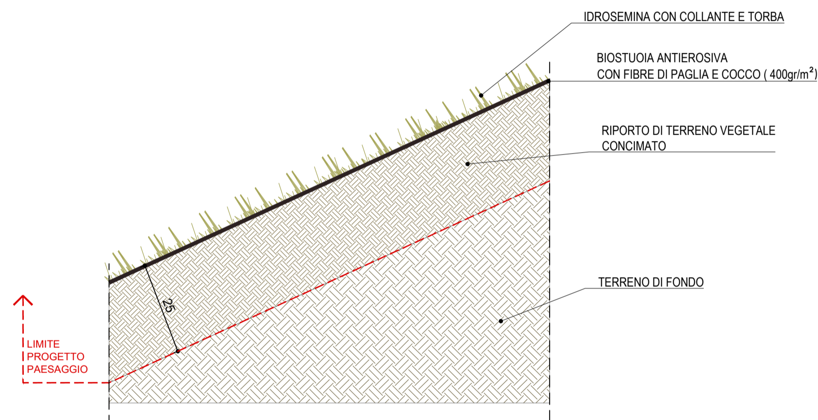
04 PRATO RUSTICO SU SCARPATA 1:10
