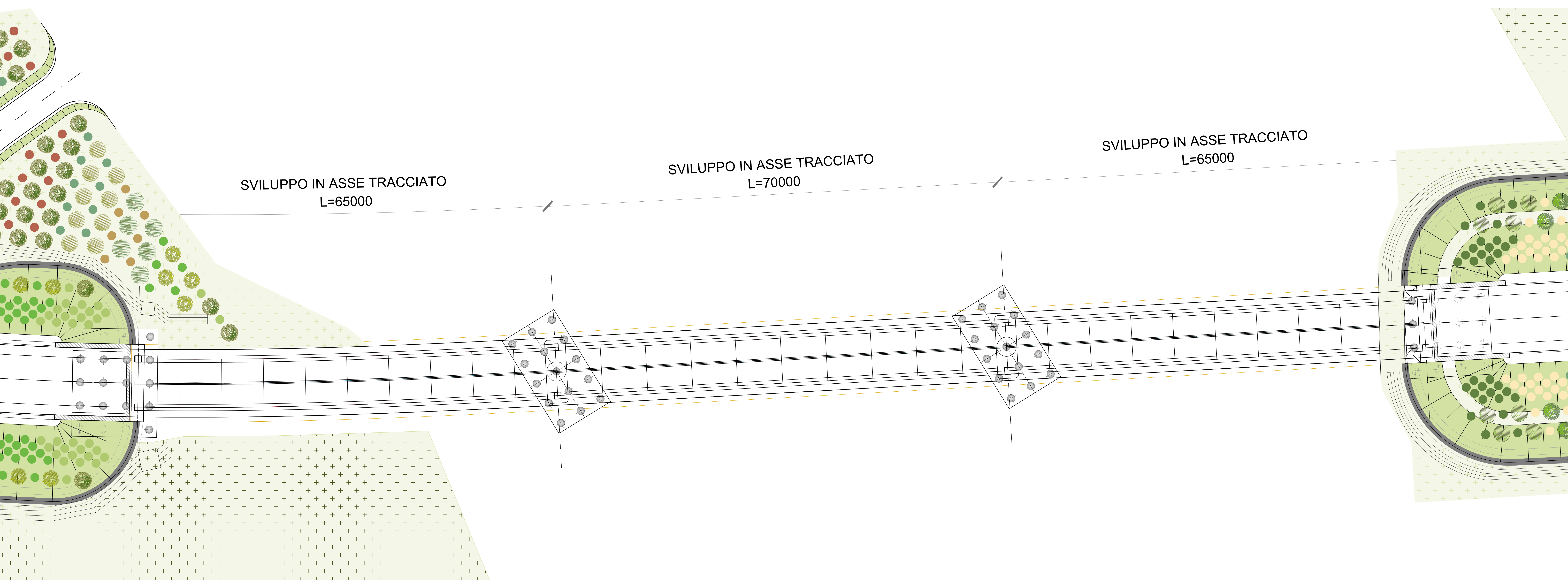
01 STRALCIO PLANIMETRICO VIADOTTO SU Fiume TORDINO 1:200
