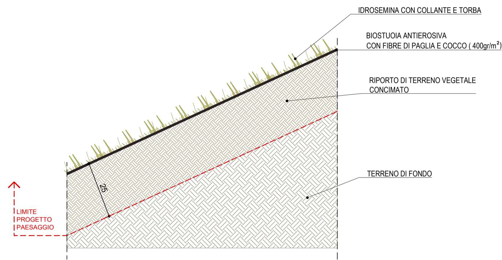
04 PRATO RUSTICO SU SCARPATA 1:10
