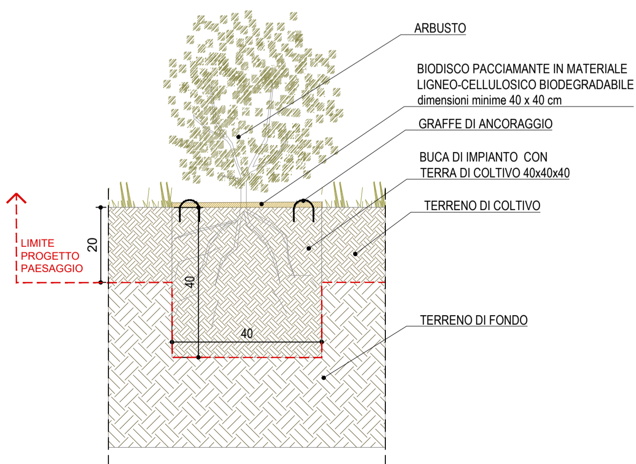
06 ARBUSTO IN PIENA TERRA 1:10
