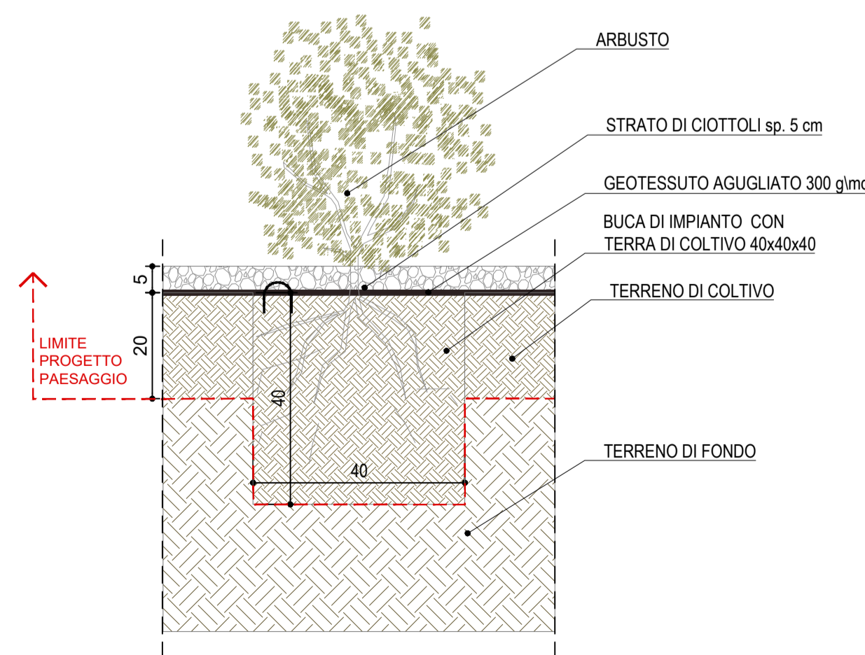
07 ARBUSTO SU GHIAIA 1:10
