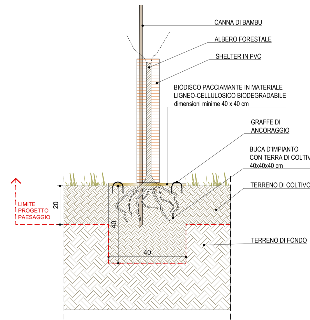
05 ALBERO FORESTALE 1:10
