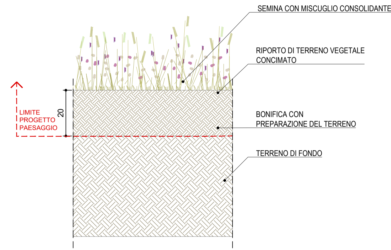
02 RINVERDIMENTO RIPRISTINO AREE CANTIERE - PRATO RUSTICO 1:10
