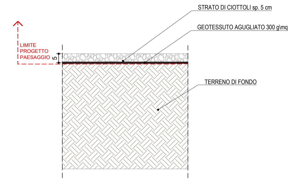
03 PAVIMENTAZIONE IN GHIAIA 1:10
