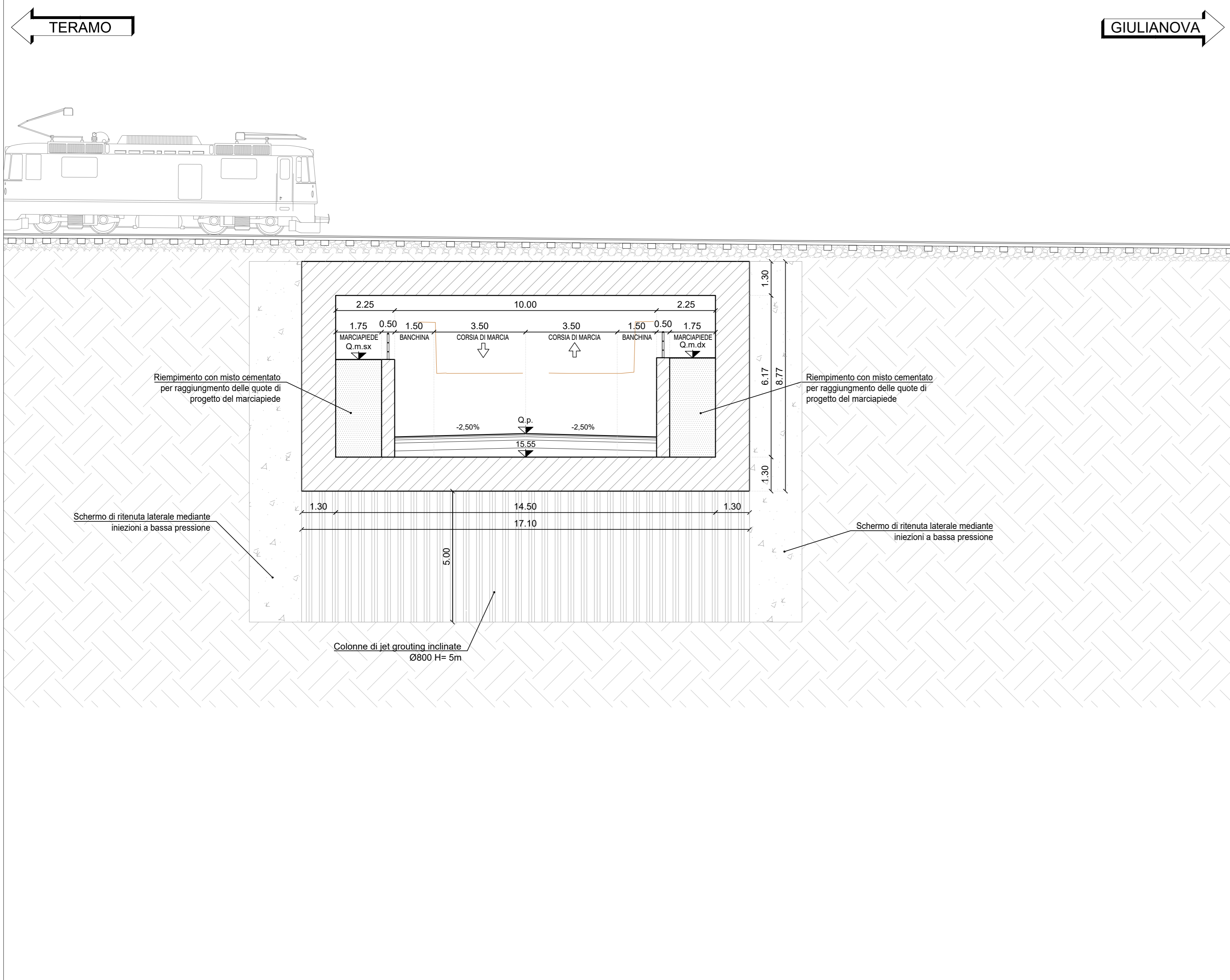
SEZIONE TIPOLOGICA C-C SCALA 1:100
