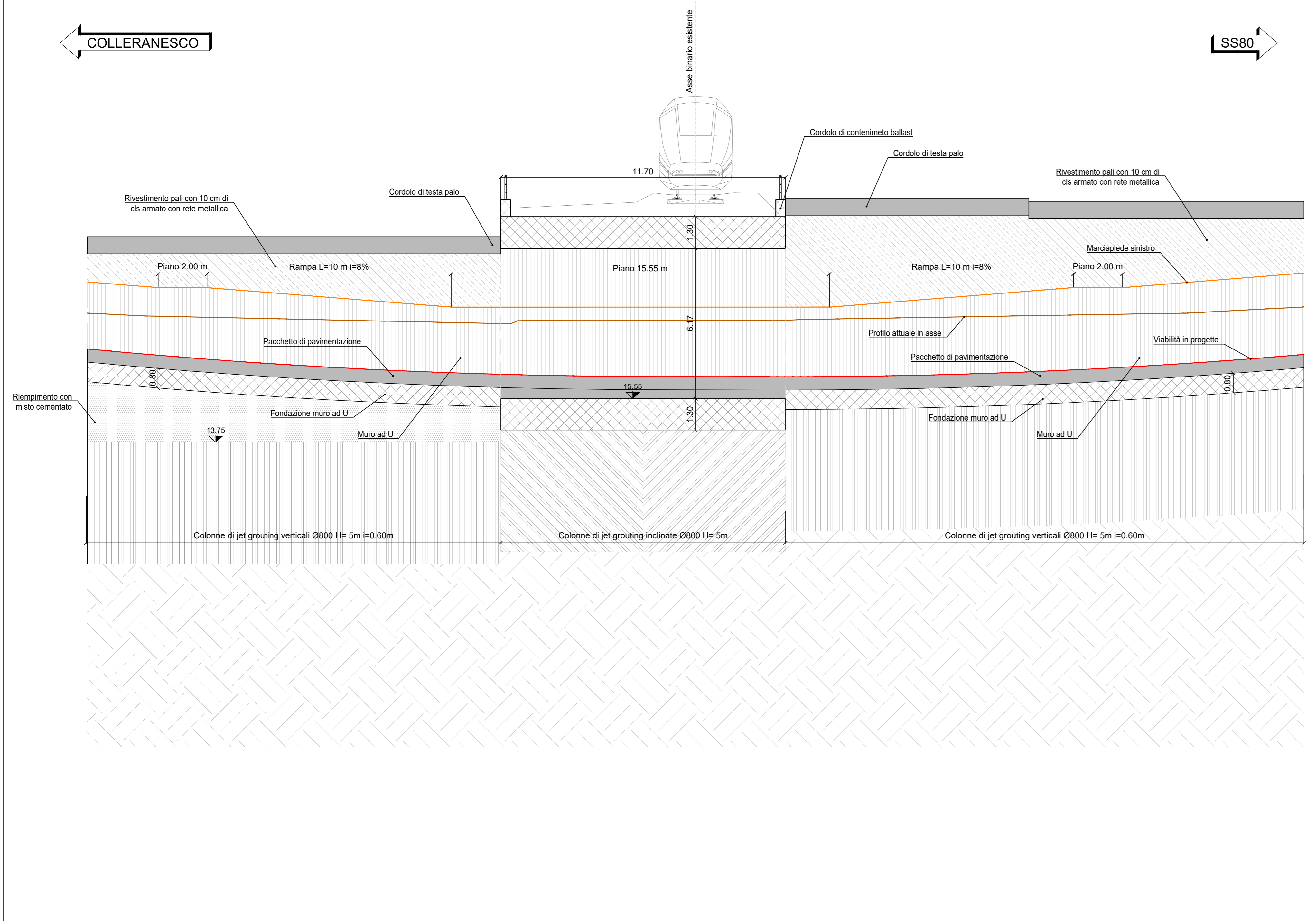
SEZIONE TIPOLOGICA C-C SCALA 1:100
