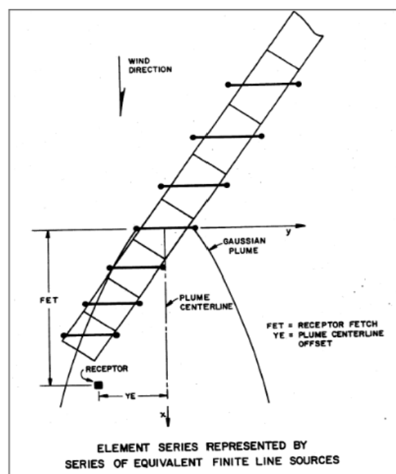
Trattamento della sorgente lineare in CALINE 4
