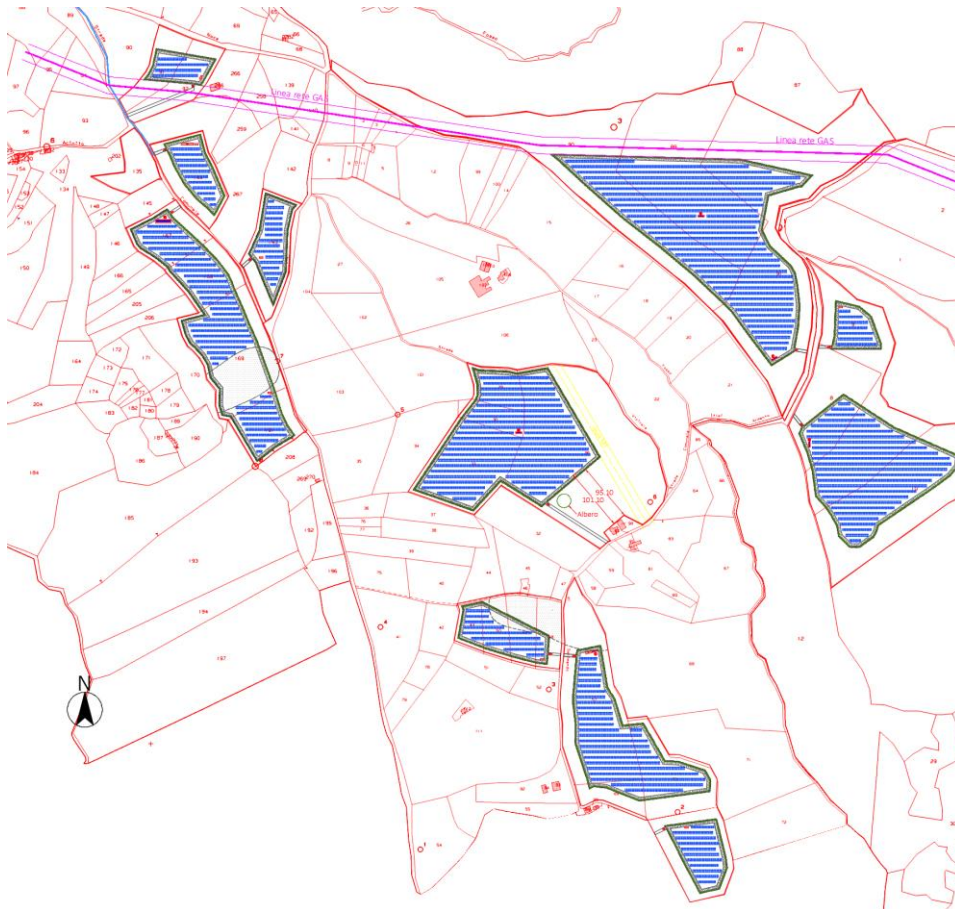
Planimetria generale impianto fotovoltaico (stralcio dalle tavole di progetto)
