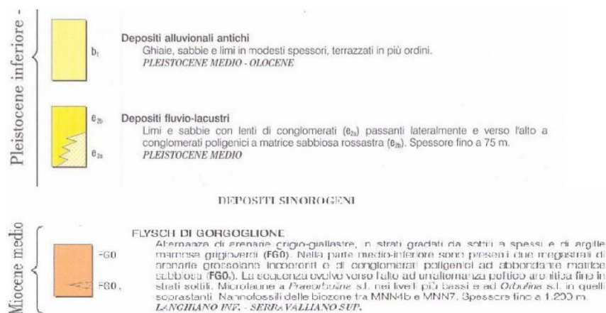
Figura 5: Stralcio del Foglio N. 506 della Carta geologica d'Italia Scala 1:50.000
