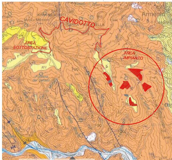
Figura 5: Stralcio del Foglio N. 506 della Carta geologica d'Italia Scala 1:50.000
